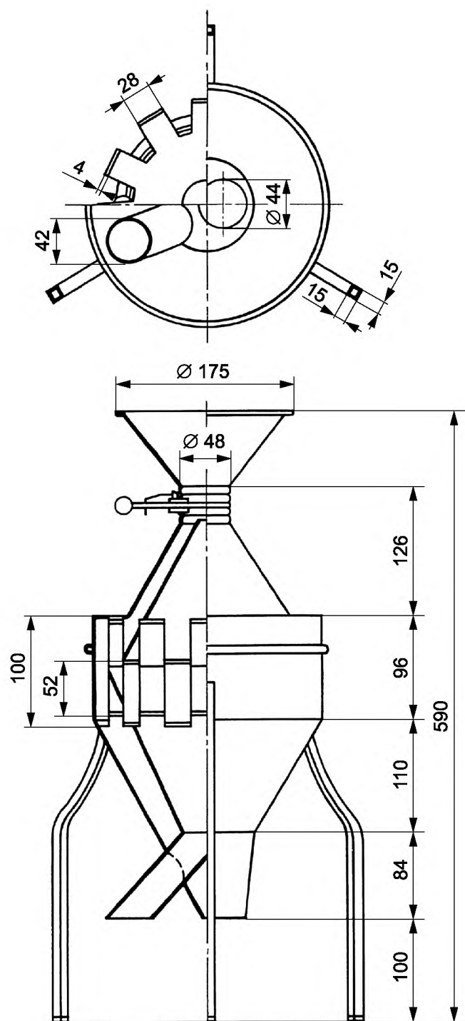
Рисунок 2 — Конический делитель
