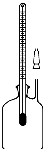
Рисунок 1 — Пикнометр Джолмеса
