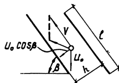
Рис.2. Схема движения частицы в наклонной ячейке
