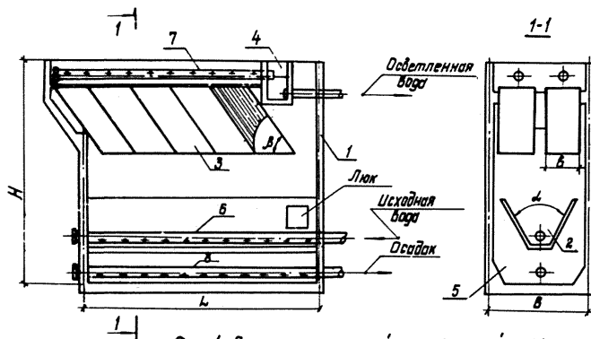
Рис.1. Схема тонкослойного отстойника
