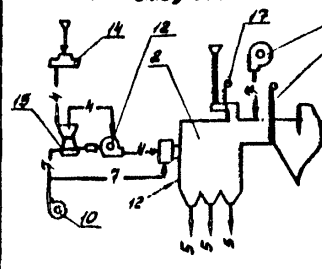
Рис. 8.4. Технологическая схема сушильной установки (барабанная сушилка) с различными типами топочных устройств.
