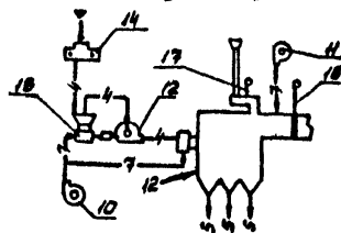
Рис. 2 Технологическая схема сушильной установки (печи) с различными типами топочных устройств.
