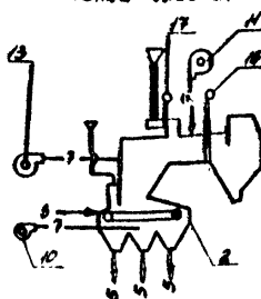
Рис. 8.4. Технологическая схема сушильной установки (барабанная сушилка) с различными типами топочных устройств.
