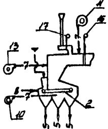
Рис. 8.3 Технологическая схема сушильной установки с трубой-сушилкой и различными типами топочных устройств.
