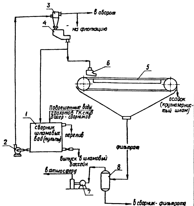
1-сборник, 2-насос, 3-гидроциклон, 4-распределительное устройство, 5- вакуум-фильтр ленточный, 6- загрузочный поток. 7- вакуум-насос, 8- ресивер.
