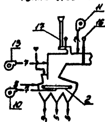
Рис. 2 Технологическая схема сушильной установки (печи) с различными типами топочных устройств.
