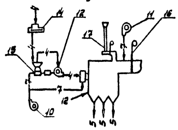
Рис. 8.3 Технологическая схема сушильной установки с трубой-сушилкой и различными типами топочных устройств.
