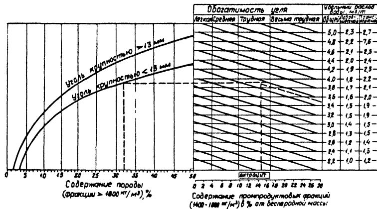
Рис. 7.Н. Номограмма для определения удельного расхода воды на отсадку угля.
