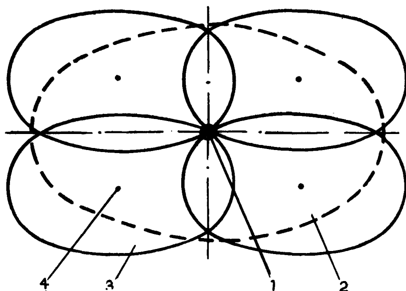
Рис. 8. Схема определения количества точек нагнетания (тампонажных скважин) на примере расчета параметров формирования изоляционной завесы в интервале водоносного горизонта 681—717 м:
