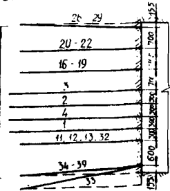
Данные о шпурах и зарядах
