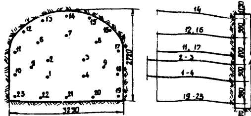
Схема расположения шпуров
