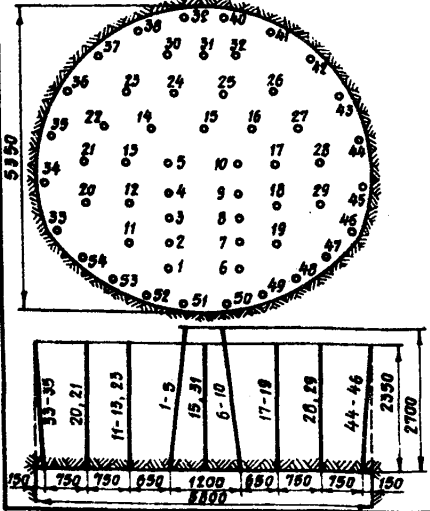
Схема расположения шпуров
