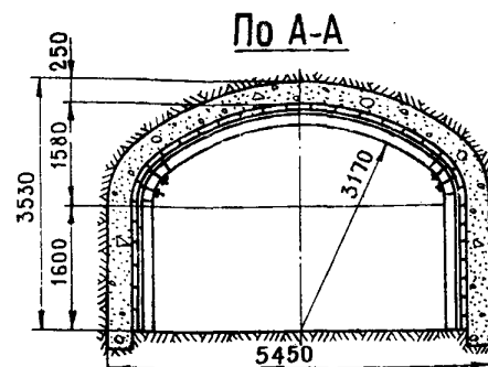
Проектное сечение
