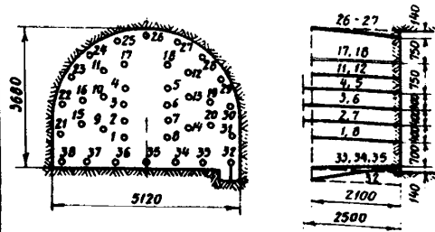
Схема расположения шпуров
