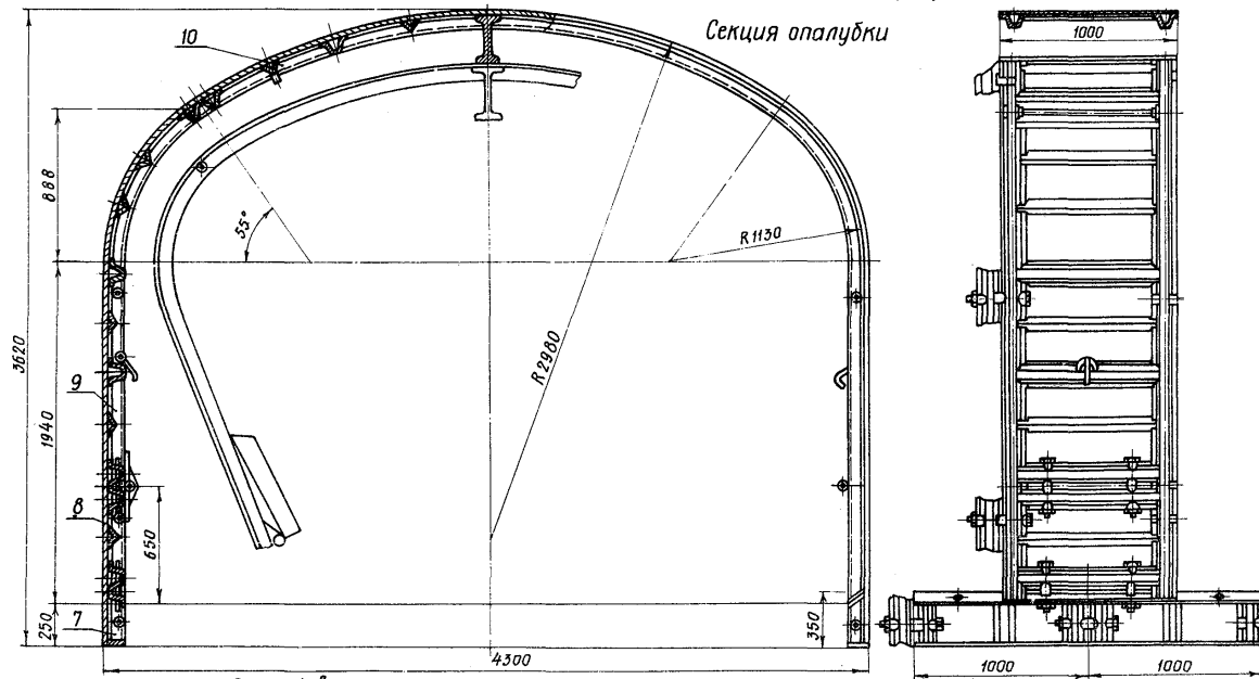
Общий вид
