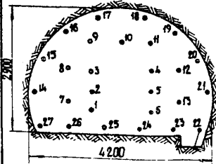
Схема расположения шпуров
