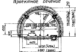
Проектное сечение
