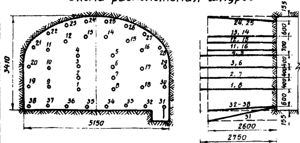
Схема расположения шпуров
