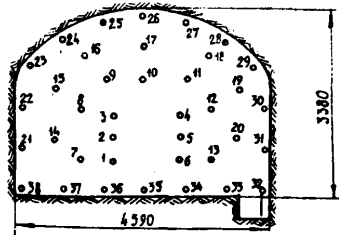
Схема расположения шпуров
