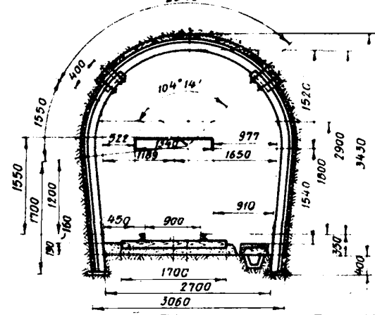
Проектное сечение 2040
