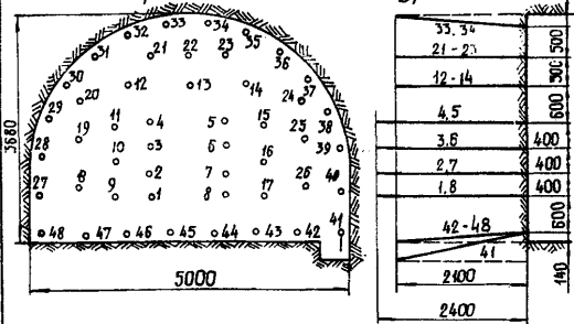
Схема расположения шпуров.
