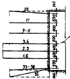
Данные о шпурах и зарядах
