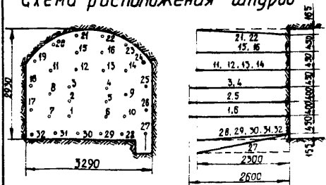
Схема расположения шпуров
