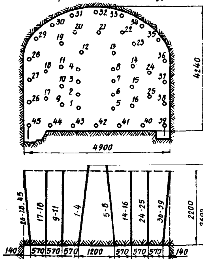
Схема расположения шпуров
