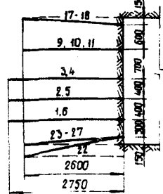
Схема расположения шпуров
