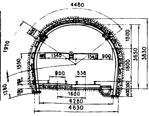
Проектное сечение
