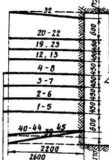
Данные о шпурах и зарядах
