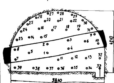
Схема расположения шпуров
