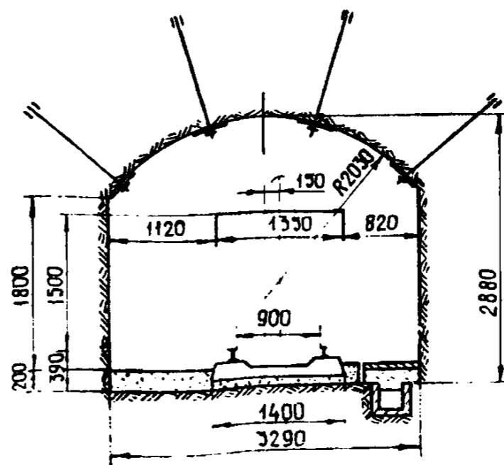
Проектное сечение
