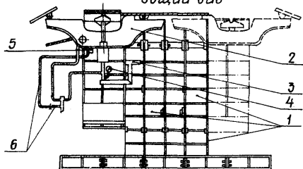
Общий вид
