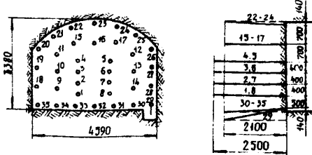
Схема расположения шпуров
