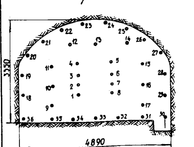
Схема расположения шпуров
