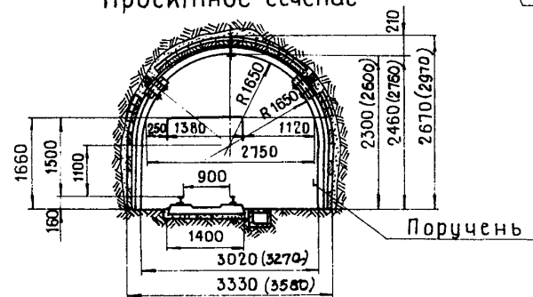
Проектное сечение
