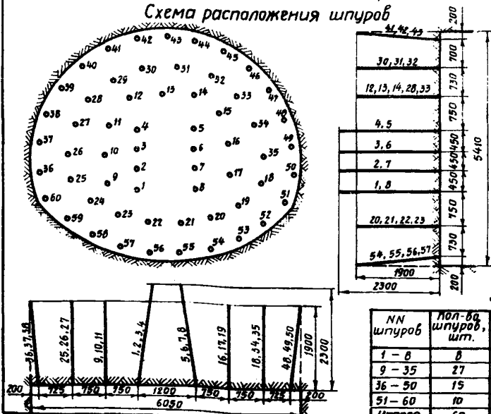
Данные о шпурах и зарядах
