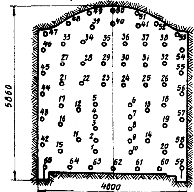
Схема расположения шпуров
