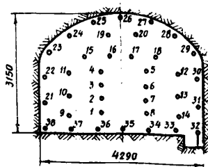
Схема расположения шпуров
