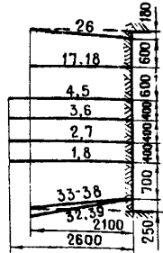
Схема расположения шпуров
