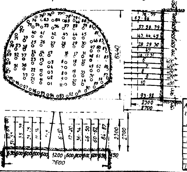
Схема расположения шпуров
