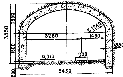
Проектное сечение
