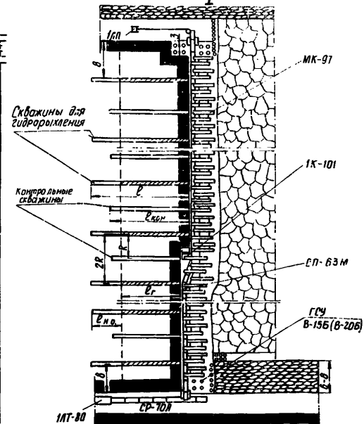
Схема очистного забоя с комплексом КМК-97
