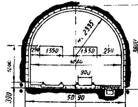
Откаточный штрек
