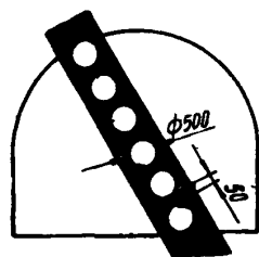
Схема раскладки скважины для выбуривания (длина 2 м)
