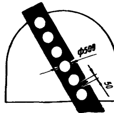
Схема расположения скважин для выбуривания (длина 2м)
