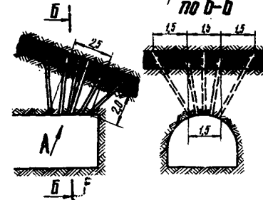
по Б-Б
