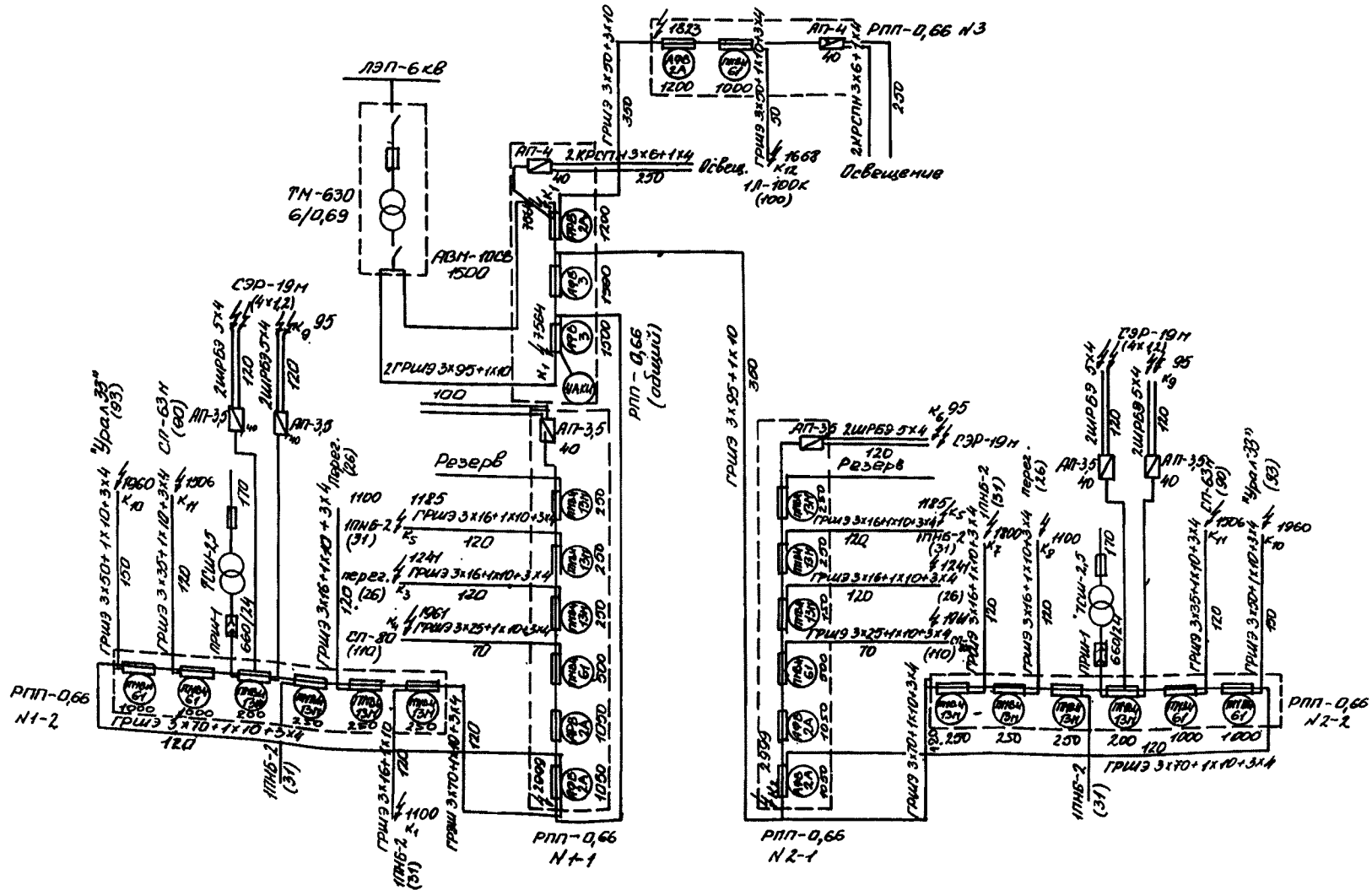
СХЕМА ЭЛЕКТРОСНАБЖЕНИЯ КАМЕРНОГО БЛОКА НАПРЯЖЕНИЕМ 660 В ПРИ КОНВЕЙЕРНОМ ТРАНСПОРТЕ (I вариант схемы очистного забоя).
