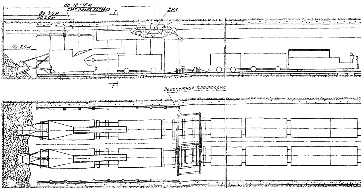
Характеристика выработки
