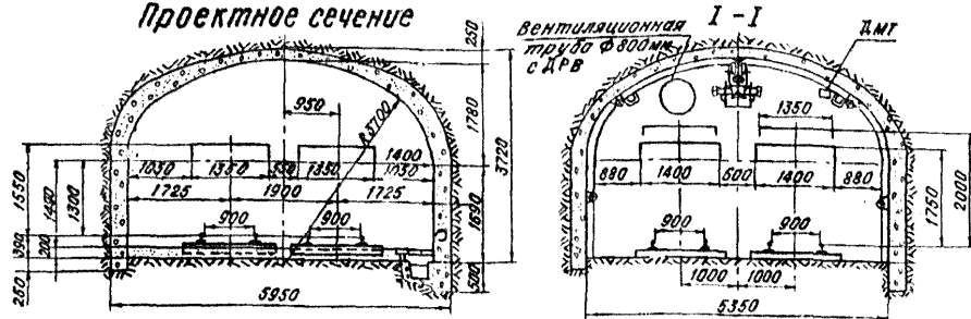
Характеристика выработки
