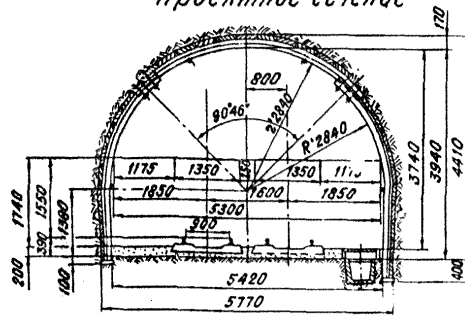
Проектное сечение
