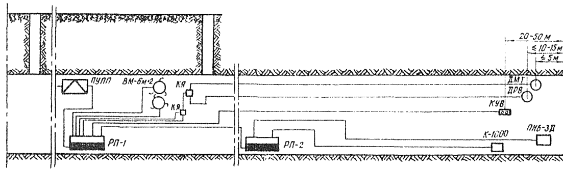
Схема электроснабжения и расстановки электрооборудования в выработке
