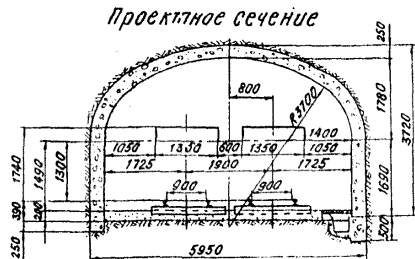
Проектное сечение
