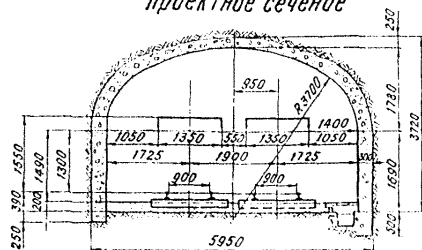
Проектное сечение
