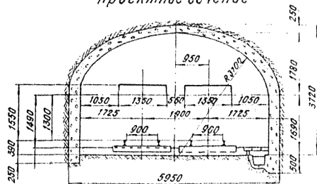
Проектное сечение
