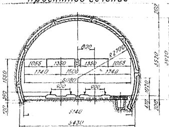
Практическое сечение
