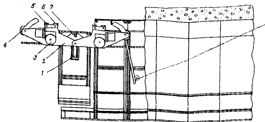
1 - домкрат; 2 - каретка; 3 - прибор; 4-6 - опорные катки; 5 - стопорное устройство; 7 - подъемная площадка; 8 - пульт управления; 9 - сводчатая часть секции; 10 - двутавр; 11 - доковая часть секции; 12 - откидная часть секции; 13 - фундаментные подставки
