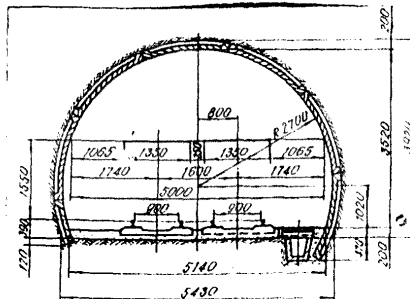
Проектное сечение
