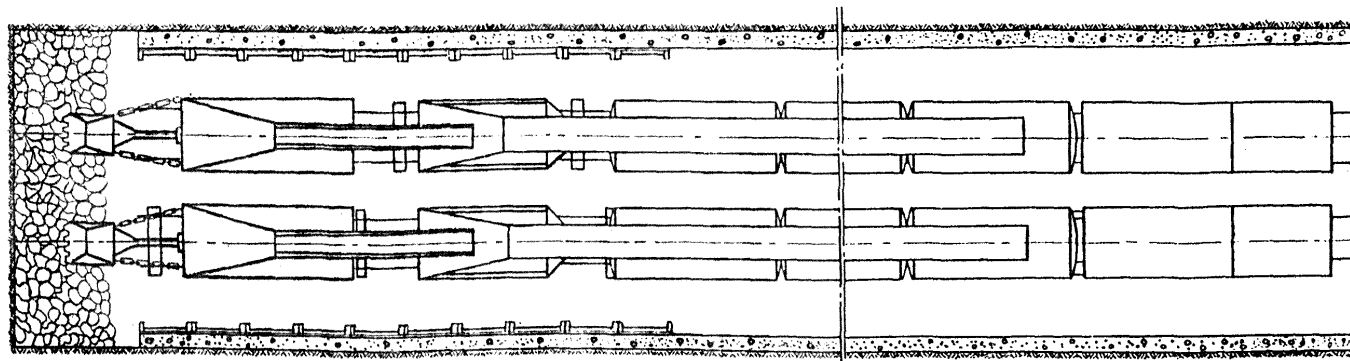
Проектное сечение
