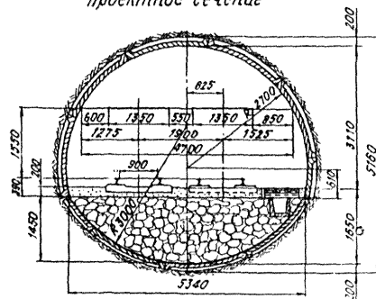
Проектное сечение
