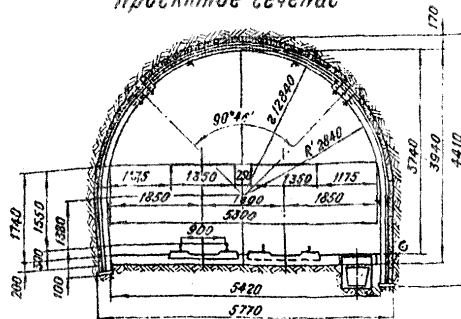
Проектное сечение
