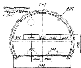
Характеристика выработки
