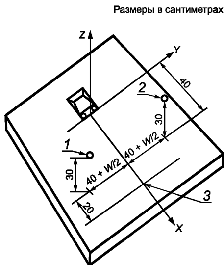
1—2 — микрофоны; 3 — конец измерения; W — ширина игрушки
