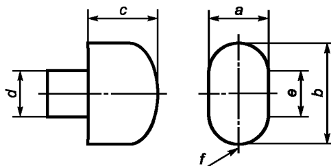
Рисунок А.1 — Щуп, имитирующий голову (для детей в возрасте младше 3 мес)
