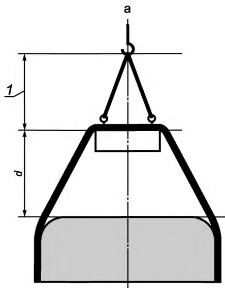
Рисунок 45 — Измерение расстояния d для игрушек с плоской поверхностью
