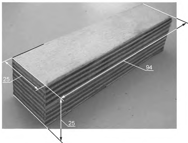
Рисунок 40 — Размеры испытательных блоков
