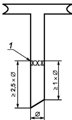
1 — постоянная метка
