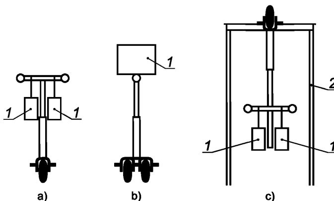
1 — испытательный груз; 2 — испытательный стол
