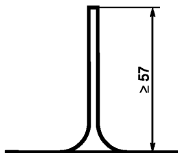
Рисунок 13 — Измерение длины снаряда с вакуумной присоской
