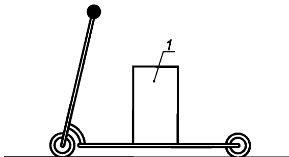
1 — испытательный груз
