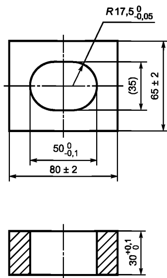
Рисунок 24 — Испытательный шаблон А
