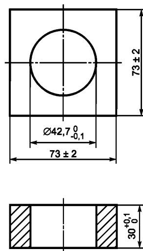
Рисунок 25 — Испытательный шаблон В
