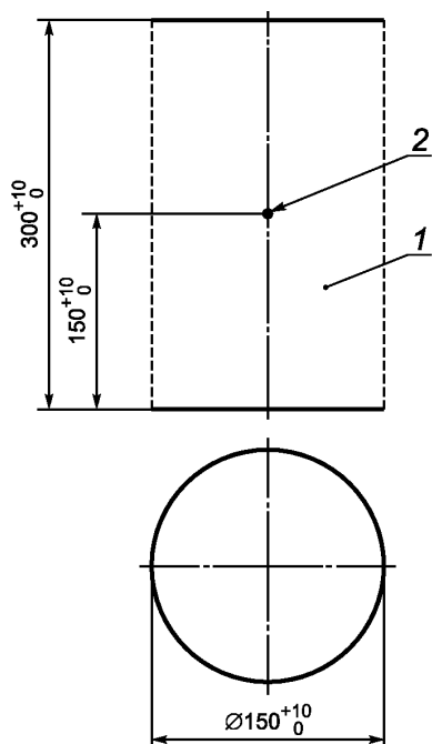
Рисунок 26 — Испытательные грузы для определения прочности и устойчивости
