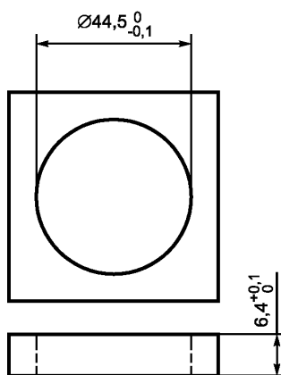
Рисунок 37 — Испытательный шаблон Е
