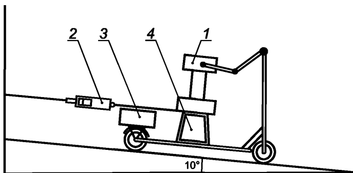
1 — испытательная нагрузка, с шарнирным рычагом — (25 \pm 0,5) кг на каждый рычаг; 2 — динамометр; 3 — испытательная нагрузка, (25 \pm 0,5) кг; 4 — платформа и стабилизирующее устройство высотой 250 мм и массой (4,8 \pm 0,2) кг
