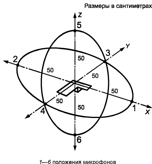
Рисунок 36 — Положения микрофонов при измерении уровней звукового давления излучения игрушек с пистонами
