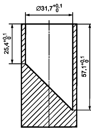
Рисунок 18 — Цилиндр для мелких деталей
