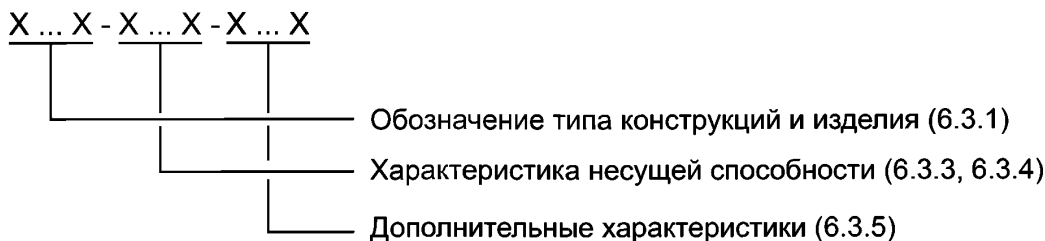
Рисунок 2 — Структура марки типовых конструкций в чертежах КМ
