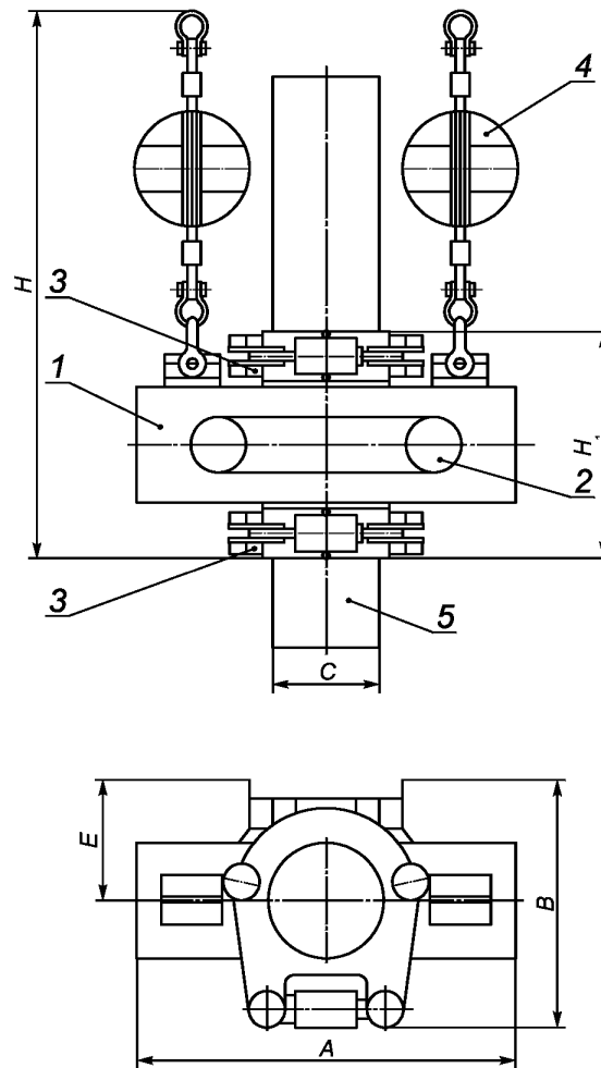
Рисунок А.14 — Вибропогружатели с гидравлическим приводом для погружения забивных труб
