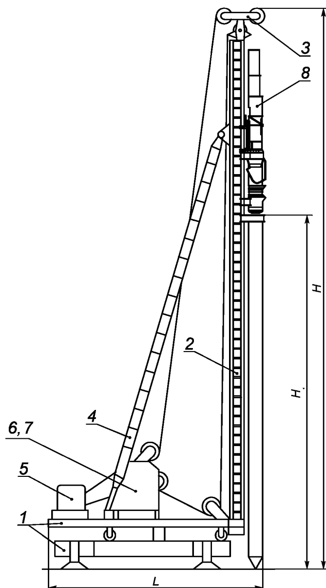
1 — рельсовое ходовое устройство; 2 — погружатель, установленный непосредственно на ходовое устройство; 3 — оголовок мачты стрелы погружателя; 4 — раскос; 5 — привод; 6 — лебедка управления свай; 7 — лебедка управления сваебойным молотом; 8 — оборудование для погружения свай
