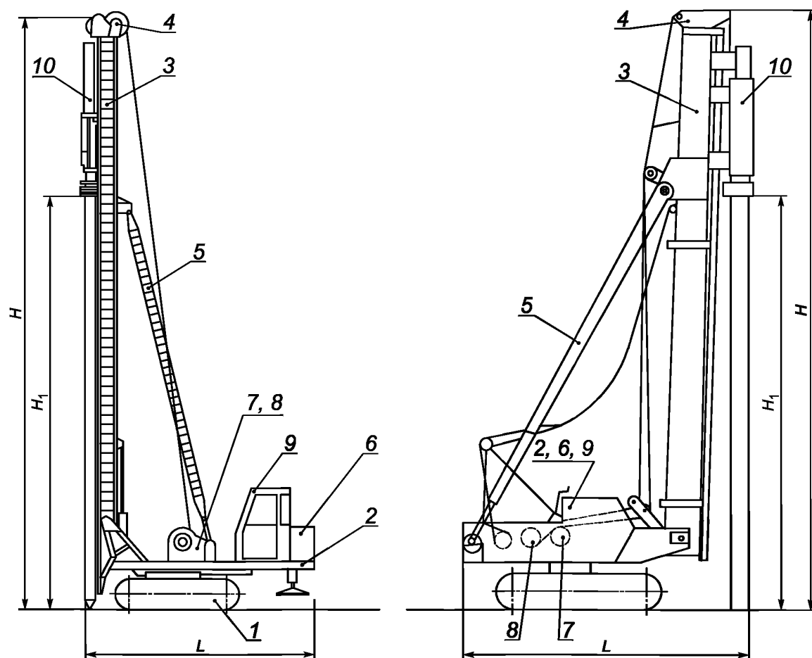
а) позиционирование сваи с помощью гидроцилиндра б) позиционирование сваи с помощью лебедки
