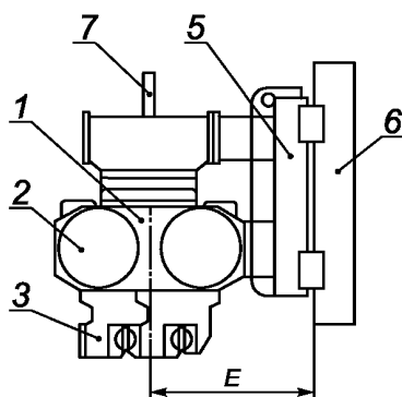
б) Вибропогружатель для установки на свайном оборудовании
