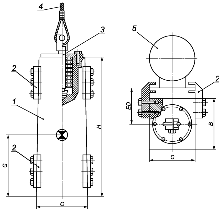
Рисунок А.8 — Механический молот с лебедкой
