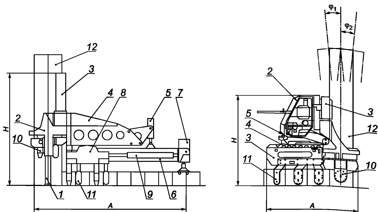
Рисунок А.15 — Оборудование для извлечения свай с пневматическим приводом ударного действия
