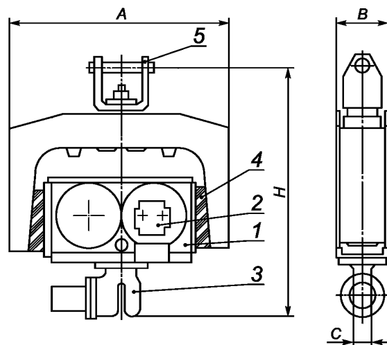
б) Вибропогружатель для установки на свайном оборудовании
