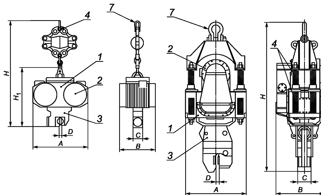
а) Вибропогружатели для грузоподъемных кранов
