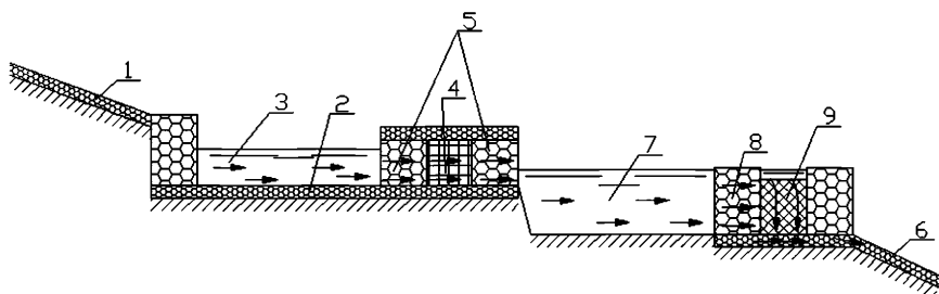
Рисунок 2 – Схема пруда-отстойника
