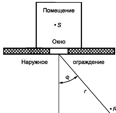
Рисунок 2 — Схема для определения угла \varphi между нормалью к наружному ограждению и направлением в расчетную точку
