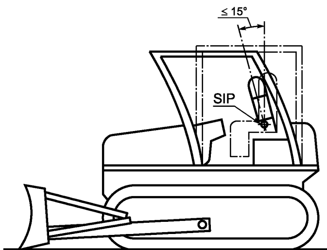
б) Продольная нагрузка на бульдозер
