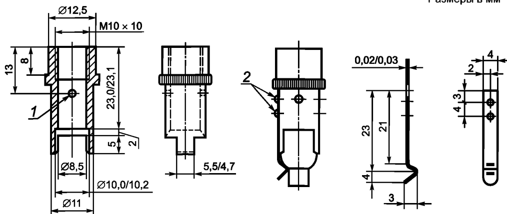
Рисунок 5 — Корпус
