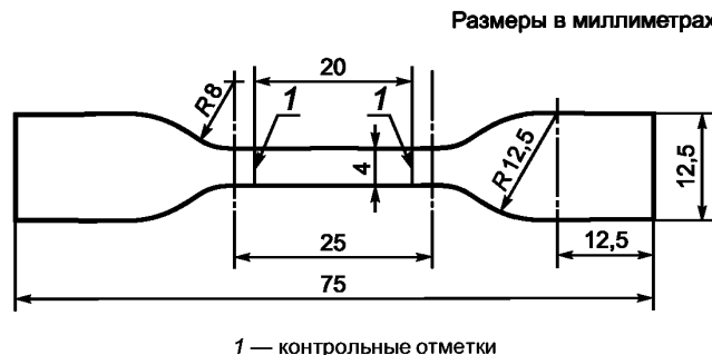
Рисунок 1 — Образец в виде двусторонней лопатки
