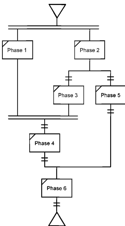
Рисунок 36 — Некорректная процедурная функциональная диаграмма
