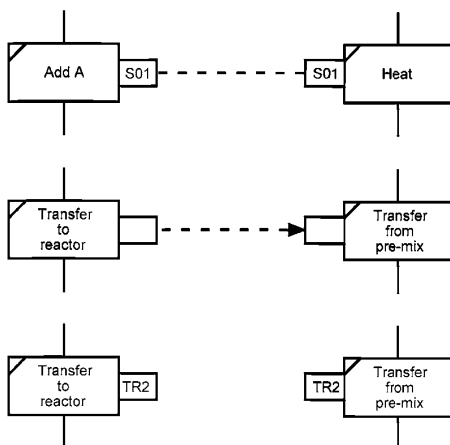
Add A — добавить компонент а; heat — нагрев; transfer to reactor — передача материала в реактор; transfer from pre-mix — передача после предварительного смешивания
