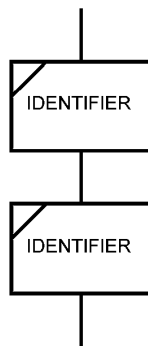
Рисунок 27 — Неявный переход
