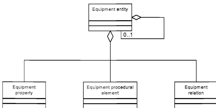
Рисунок 8 — Структура оборудования
