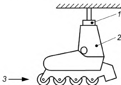
1 — колодка; 2 — роликовый конек; 3 — направление удара
