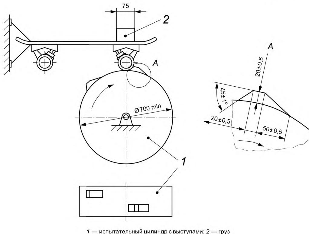
Рисунок 4 — Испытание износостойкости скейтборда
