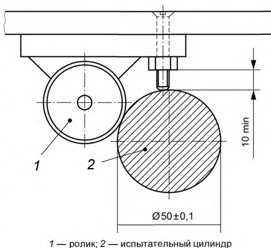
Рисунок 5 — Испытание выступающих элементов подвески
