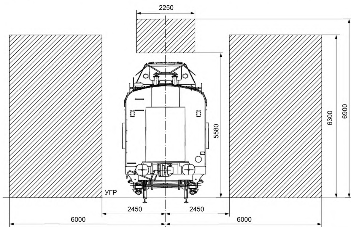
Рисунок 1 — Расположение зон, видеоизображение объектов в которых должно регистрироваться комплексами (по отношению к железнодорожному пути)
