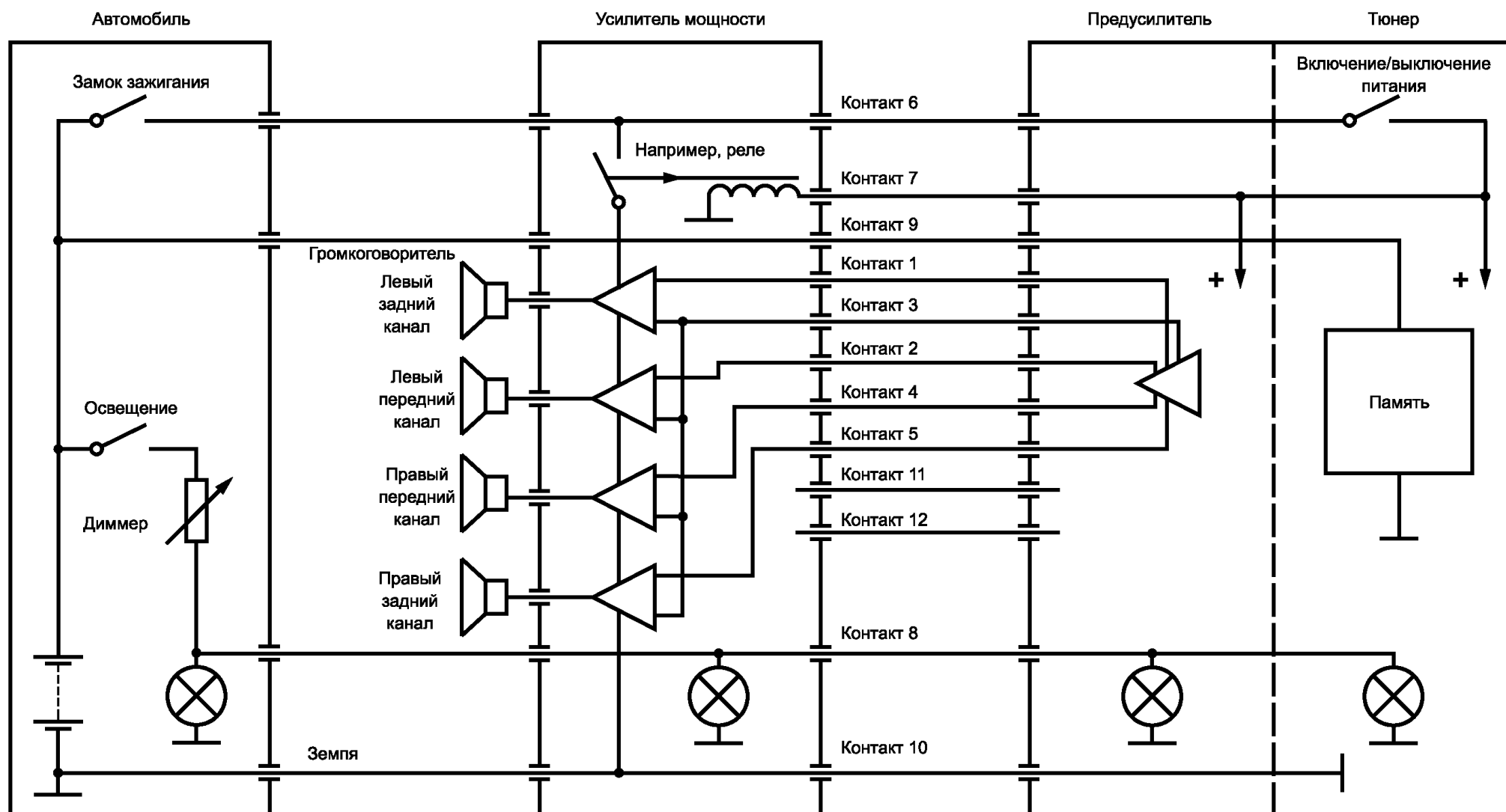
Рисунок В.2 — Схема применения 12-контактных соединителей (см. 5.15 в таблице 1В)
