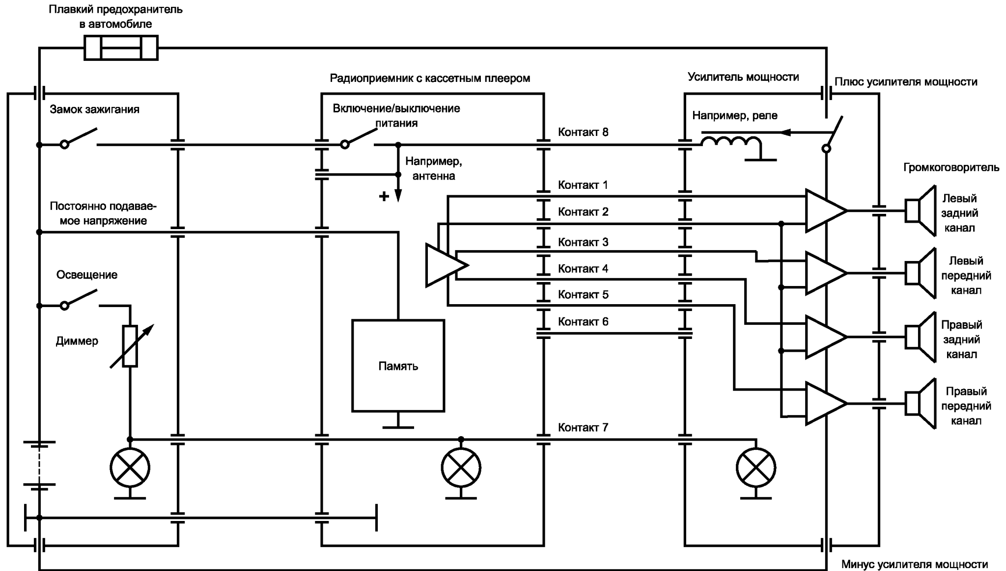
Рисунок В.1 — Схема применения 8-контактных соединителей 130-9 МЭК 20 и 21 (см. 5.14 в таблице 1В)
