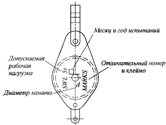
Рис. 11.2.1-5 Маркировка блока
