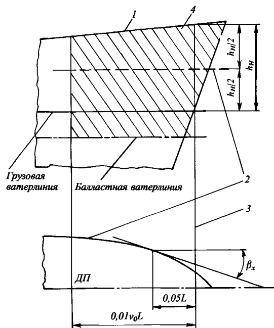
Рис. 2.8.1.2-2 Схема определения угла \beta_x и области действия ударного давления волн (заштрихована):
