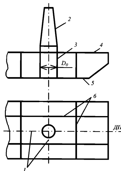
1 — переборки крестовины; 2 — неподвижная опорная колонна; 3 — барабан; 4 — верхняя палуба; 5 — днище; 6 — переборки опорного контура
