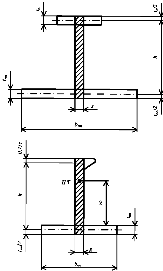
Рис. 3.10.4.2.5: — площадь, засчитываемая в фактическую площадь стенки A_{\phi}
