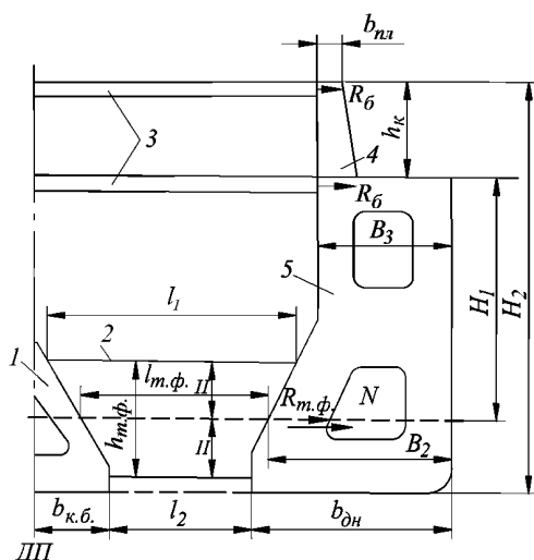
1 — килевая балка; 2 — трюмный флор; 3 — бимсы; 4 — рамная стойка комингса; 5 — диафрагма
