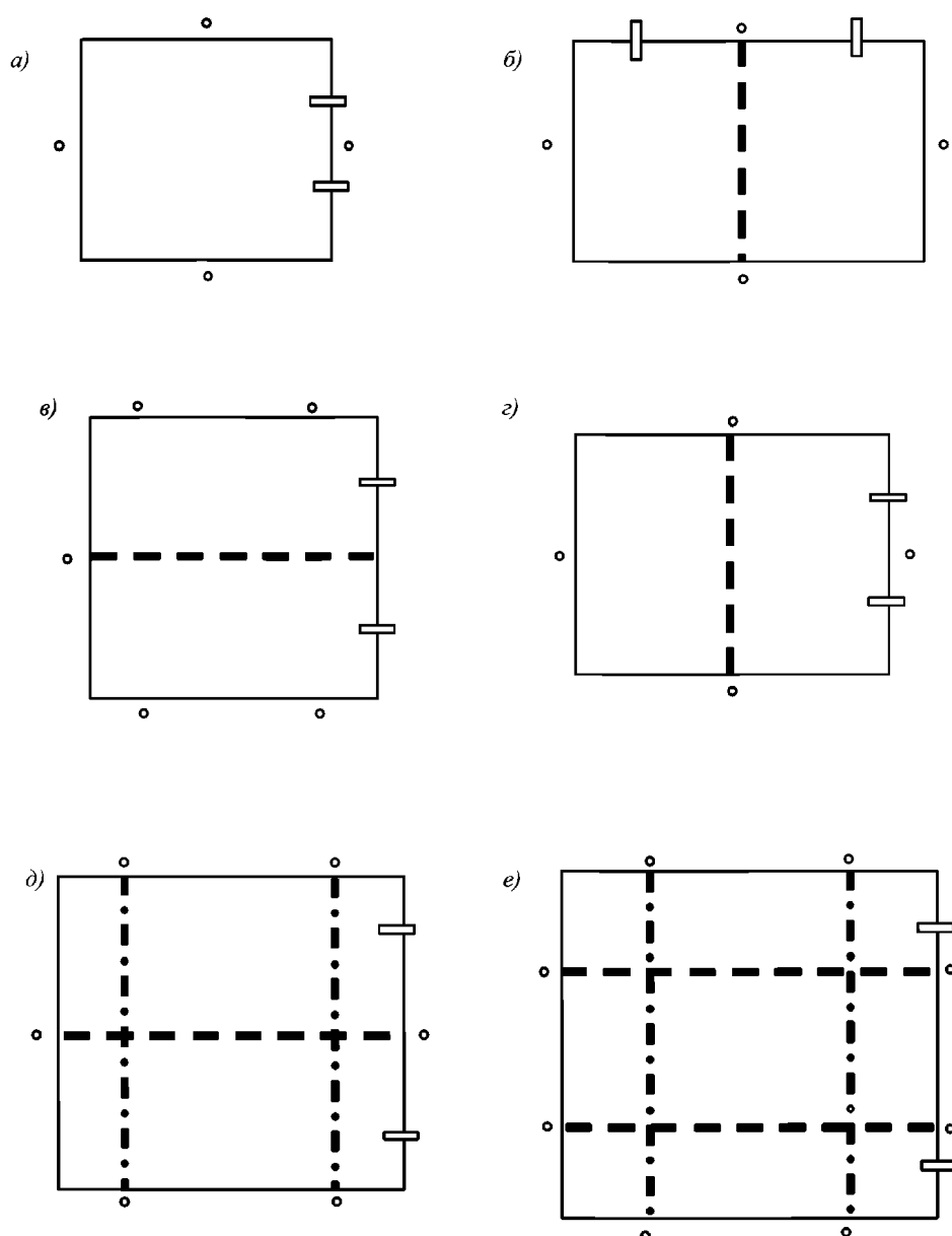
Рис. 7.7.2.2 Номинальные размеры люковых закрытий:
