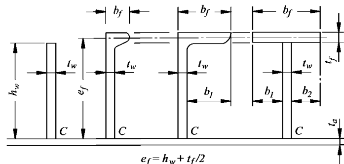
Рис. 7.10.6.31 Размеры ребра жесткости
