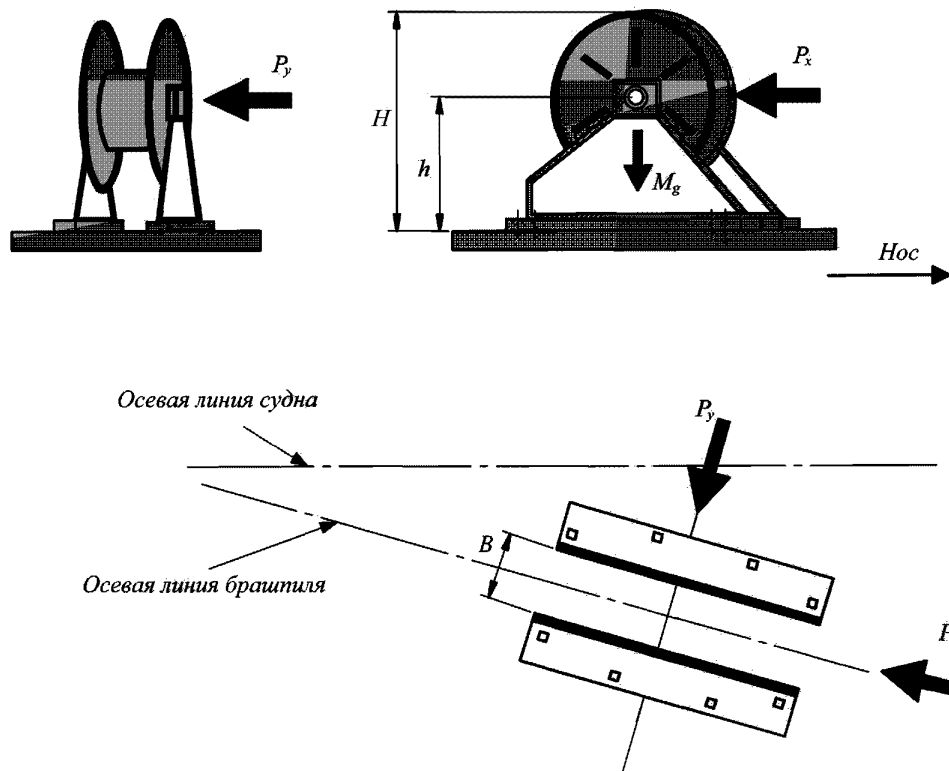
Рис. 6.3.5.3 Направление сил
