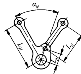
Рис. 2.4.3-2 Прицепной шатун
