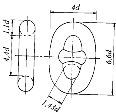
Рис. 7.1.3-2 Увеличенное звено
