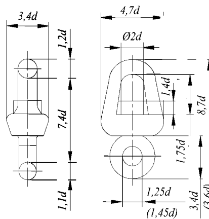
Рис. 7.1.3-7 Вертлюг
