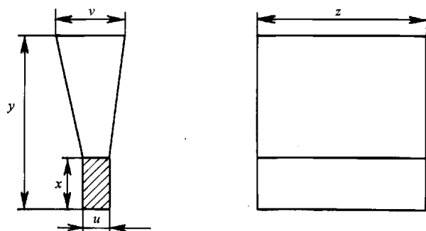
Рис. 3.9.5.1-3 Стандартный образец и альтернативные образцы с размерами:
