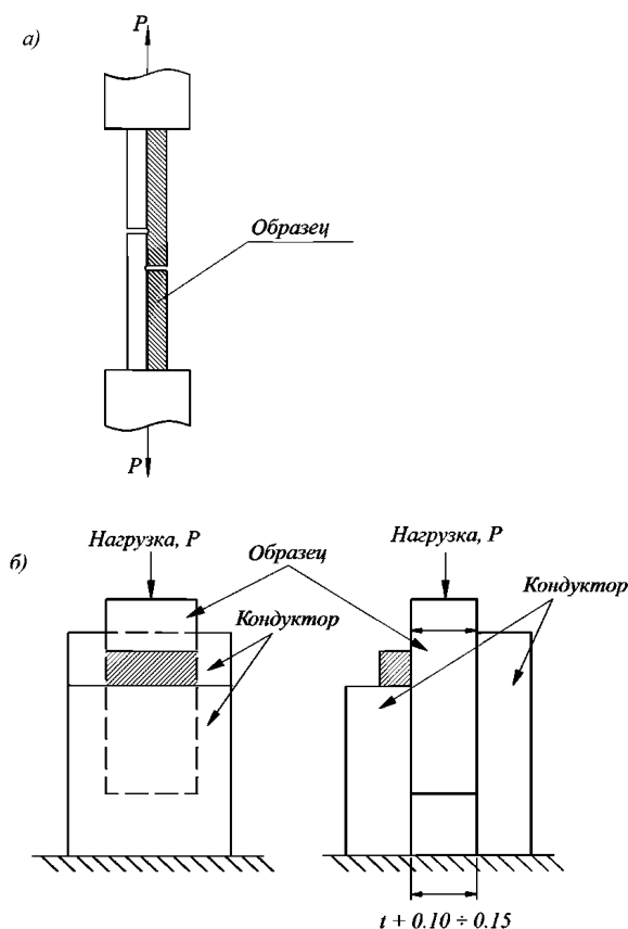
Рис. 5.3.2.3.4.3.2-2 Схемы испытания на срез (а или б)
