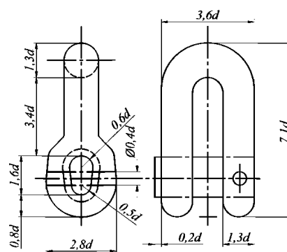
Рис. 7.1.3-5 Соединительная скоба
