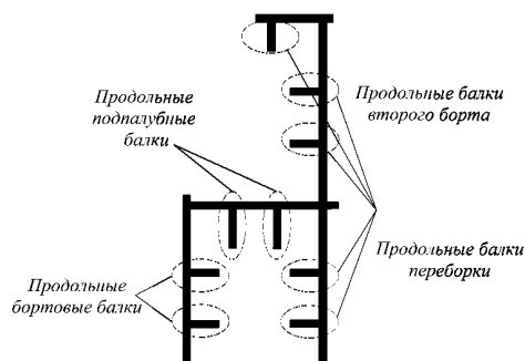
Рис. 3.20.2.1.1.1 Элементы верхнего пояса эквивалентного бруса
