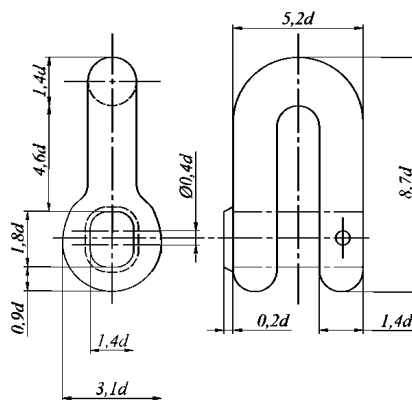
Рис. 7.1.3-6 Концевая скоба
