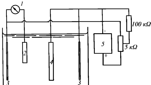
Рис. 2.5.6.1-2 Гальваностатически контролируемая катодная защитная цепь:
