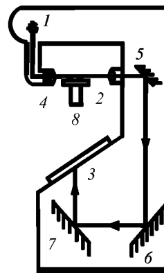
Рис. 2.5.7.2 Прибор, рекомендуемый для определения краевого угла смачивания:
