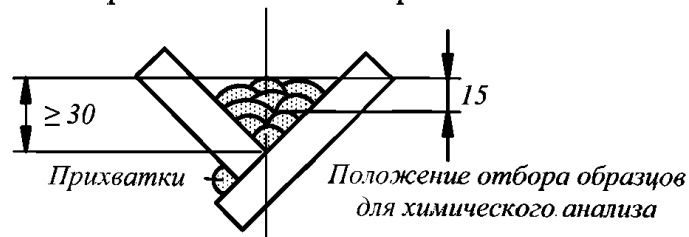
Рис. 4.10.2 Проба для испытаний наплавленного металла
