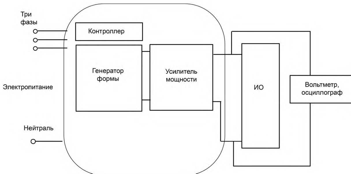
Рисунок 3 — Схема однофазного испытательного оборудования с усилителем мощности
