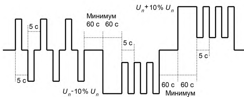
Рисунок 2 — Пример последовательного применения колебаний напряжения
