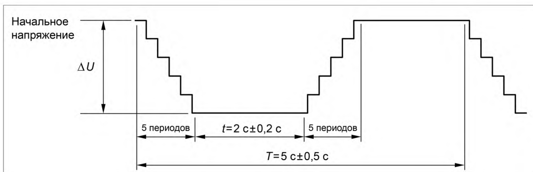
Рисунок 1d — Пример полного колебания напряжения
