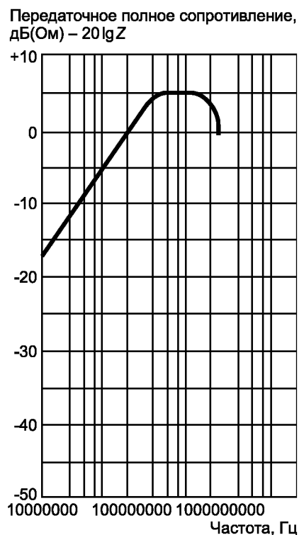
Рисунок В.3 — Передаточное полное сопротивление типовых токоёмников
