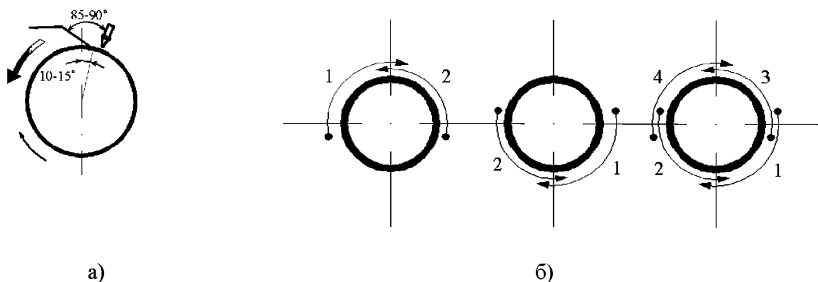
а) с поворотом на 360^\circ ; б) в два поворота на 180^\circ
