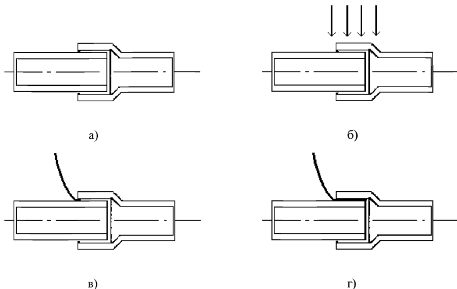
а) сборка трубы с раструбом (фитингом); б) равномерный нагрев соединения; в) подведение припоя к одной точке монтажного зазора; г) заполнение зазора припоем
