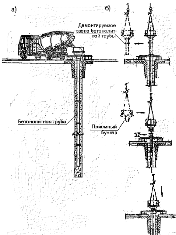
Рисунок 6.5 – Схема бетонирования
