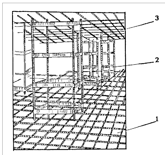
Рисунок. 5.2 – Армирование плиты (по схеме: нижняя арматурная сетка – монтажный столик – верхняя арматурная сетка)
