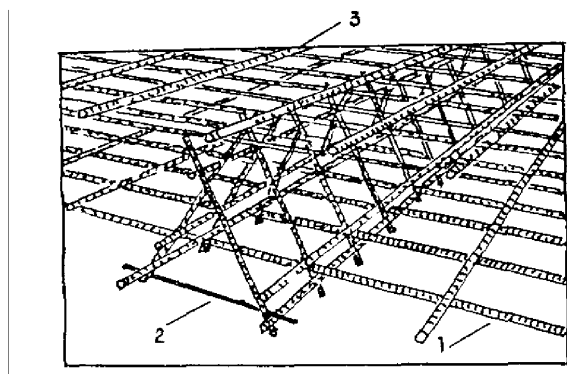
Рисунок 5.1 – Армирование плиты (по схеме: нижняя арматурная сетка – плоские или пространственные каркасы – верхняя арматурная сетка)
