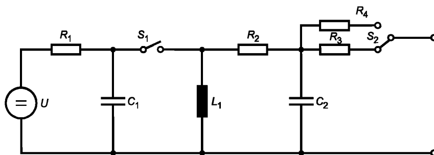
U — источник высокого напряжения; R_3 — резистор 30 Ом; C_1 — накопительный конденсатор; R_4 — резистор 12 Ом; C_2 — конденсатор фильтра; L_1 — индуктивность колебательного контура; R_1 — зарядный резистор; S_1 — высоковольтный ключ; R_2 — резистор фильтра; S_2 — селектор выходного сопротивления
