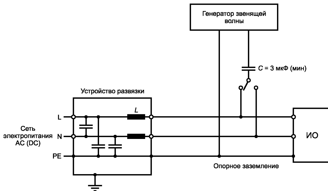
Рисунок 6 — Порт электропитания переменного или постоянного тока, однофазная сеть, испытание «линия—земля»
