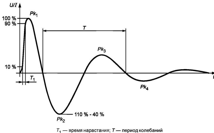
Рисунок 1 — Форма звонящей волны (напряжение холостого хода и ток короткого замыкания)
