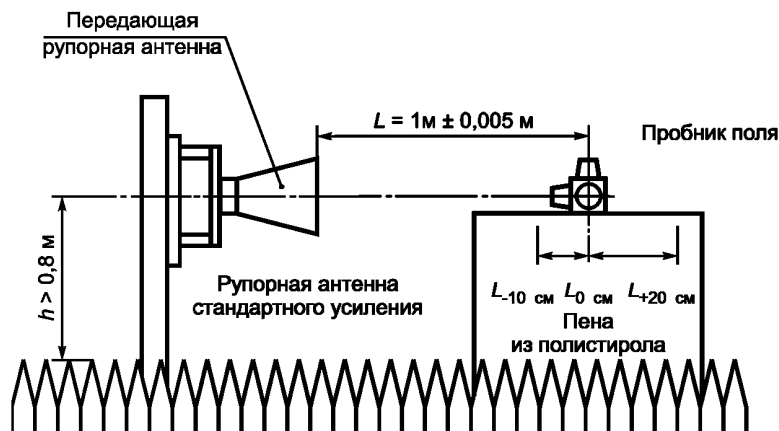
Рисунок I.3 — Испытательная установка для валидации камеры
