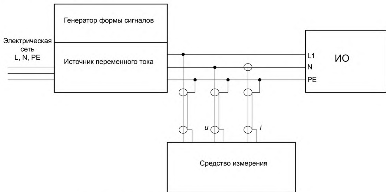
Рисунок 2 — Пример испытательной установки для однофазной сети
