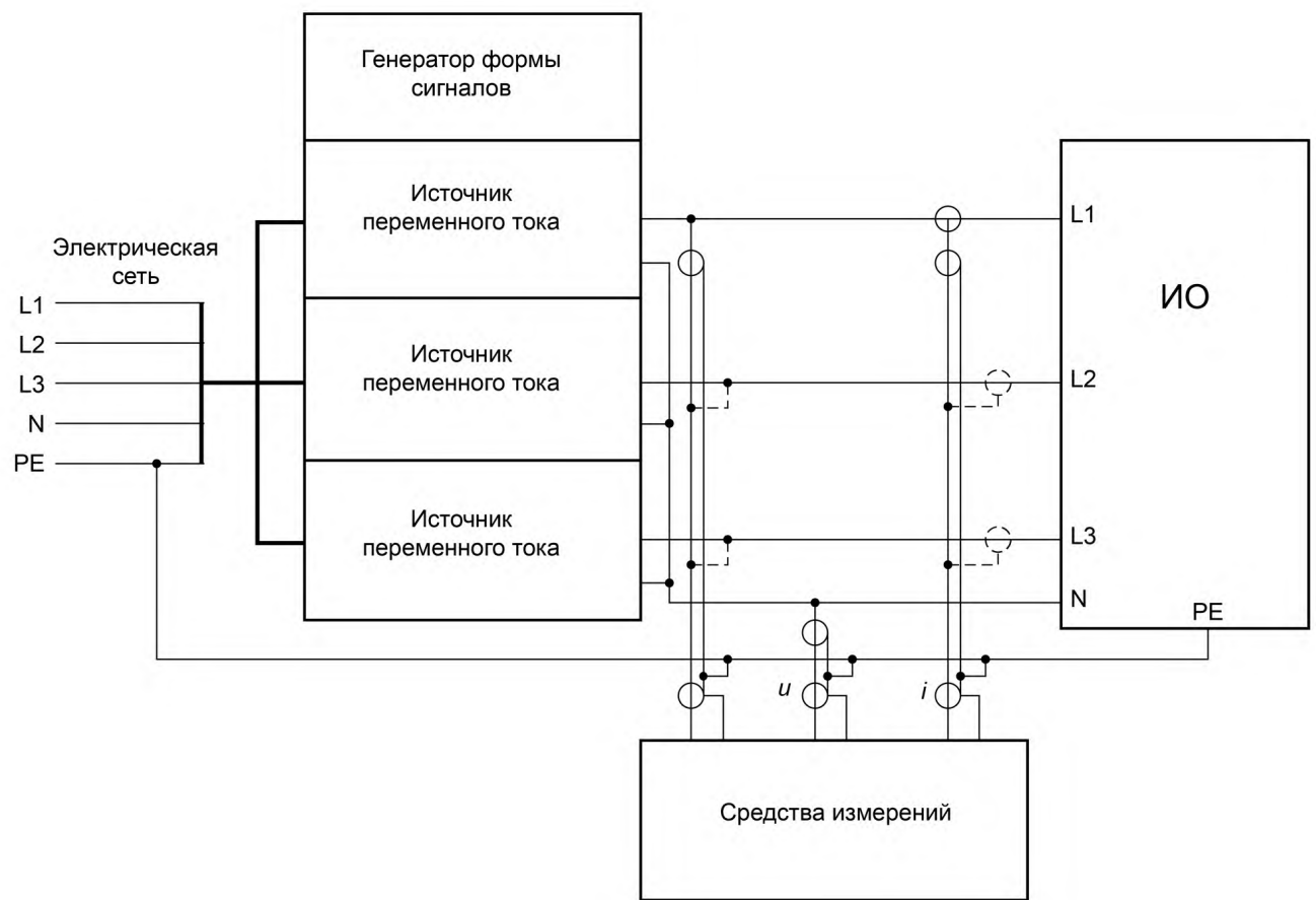
Рисунок 3 — Пример испытательной установки для трехфазной сети
