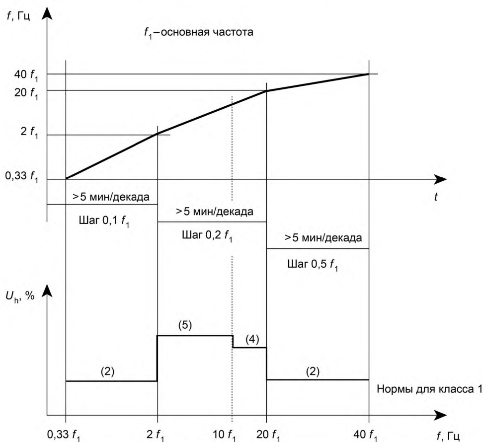
Рисунок 4 — Испытательная последовательность для отдельных гармоник
