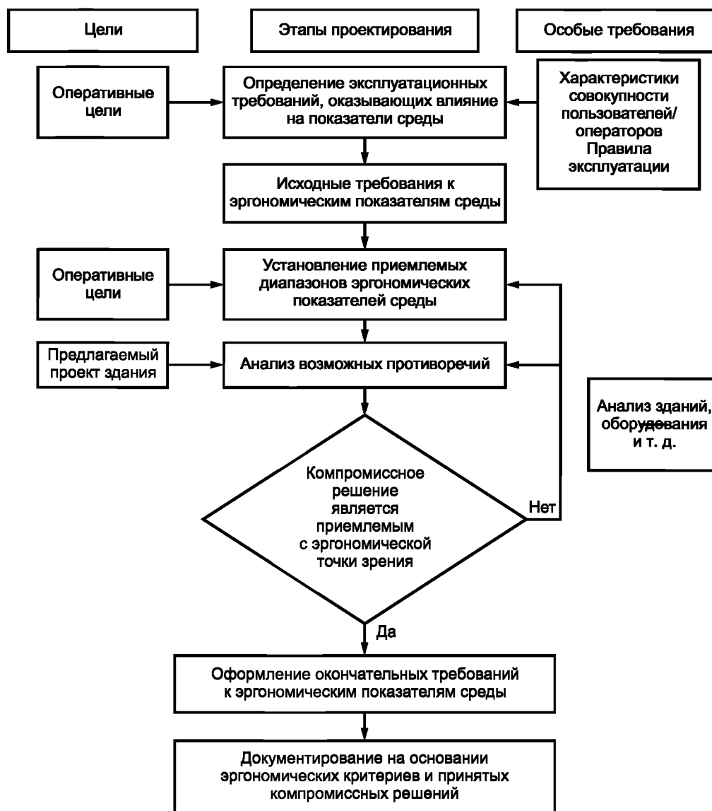
Рисунок 1 — Схема общего процесса проектирования условий окружающей среды для центра управления
