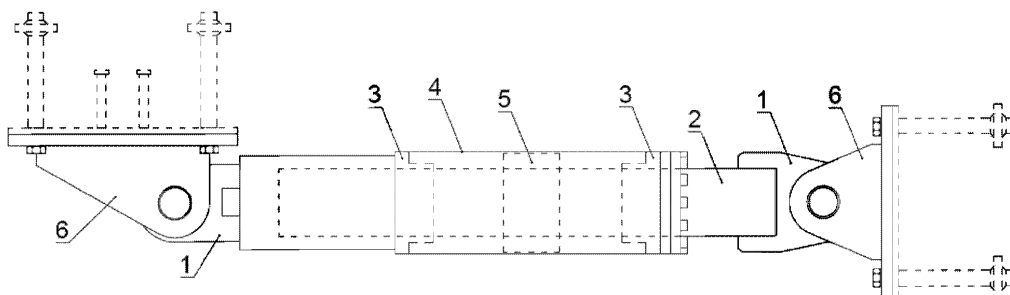
1 – шарнирный анкер; 2 – шток; 3 – крышка цилиндра с системой уплотнителей; 4 – цилиндр; 5 – поршень с системой перепуска жидкости; 6 – опорный кронштейн
