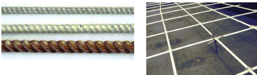
Рисунок А.1 – Общий вид стекло– и базальтокомпозитной арматуры и изготовленной из нее сетки
