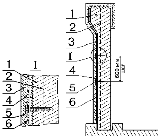
Рисунок А.17 – Подпорная стенка: 1 - усиливаемая конструкция (стена); 2 - арматура усиливаемой конструкции; 3 – торкрет-бетон усиления; 4 – полимерный органичитель; 5 – анкер; 6 - дополнительная сетка из композитной арматуры
