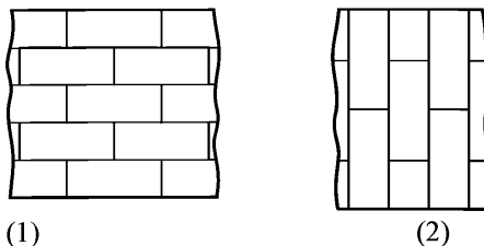
Рисунок А.2 - Варианты укладки сеток по торкретируемой поверхности: 1- укладка сеток по короткой стороне карты; 2- укладка сеток по длинной стороне карты; 3- комбинированный тип укладки карт
