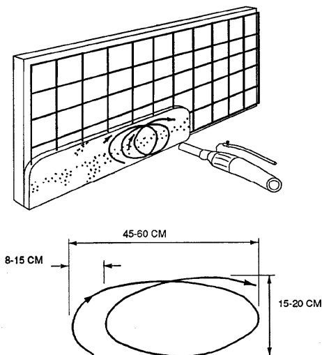
Рисунок А.7 – Схема перемещения сопла при торкретировании по композитной сетке
