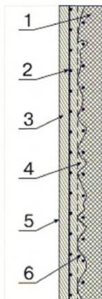
Рисунок А.15 - Восстановление бетонных поверхностей: 1 – старый бетон; 2 – арматурная композитная сетка; 3 – торкрет-бетон; 4 – восстановленный профиль; 5 – поверхность после затирки; 6 – очищенная и пескоструйно обработанная поверхность старого железобетона [7]
