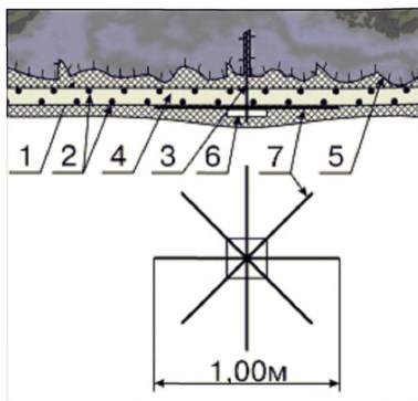
Рисунок А.14 - Армирование в области анкерной головки: 1 – торкрет-бетон; 2 – арматурная композитная сетка; 3 – анкер; 4 – слой раствора; 5 – бетонное основание; 6 – анкерная плита; 7 – двойная крестовина Ø10 мм [7]
