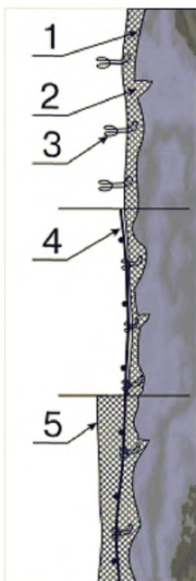
Рисунок А.5 - Крепление композитной сетки вязальной проволокой: 1 – подготовленная очищенная поверхность; 2 – торкрет-бетон; 3 – введенная в слой торкрет-бетона вязальная проволока; 4 – арматурная композитная сетка, закрепленная вязальной проволокой; 5 – выравнивающий торкрет-бетонный слой [7].
