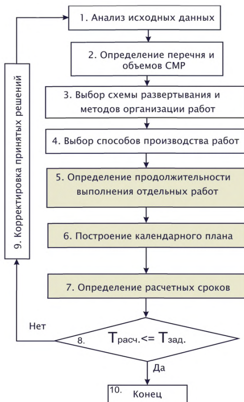
Рисунок 1 – Общая схема разработки календарного графика
