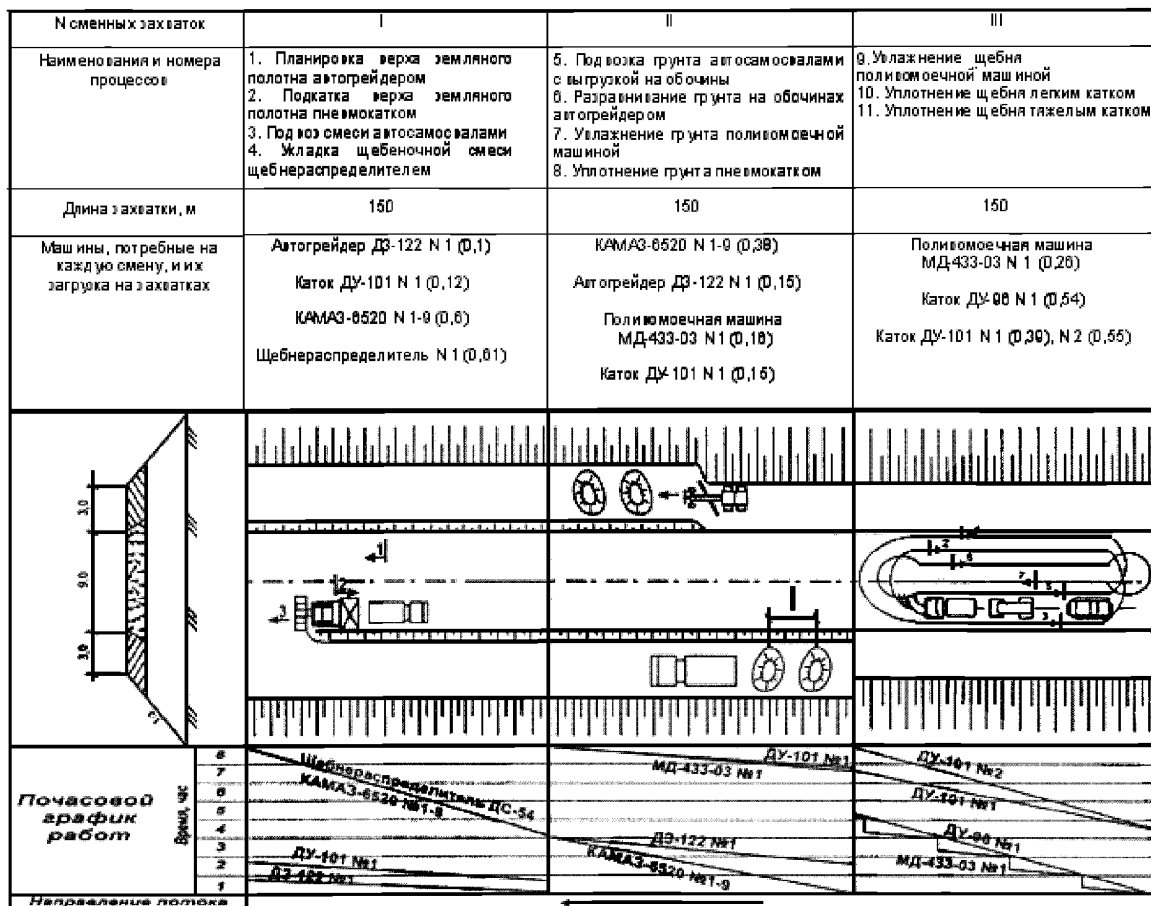
Рисунок 2 - Технологический план потока по устройству слоя основания (покрытия) из плотных смесей
