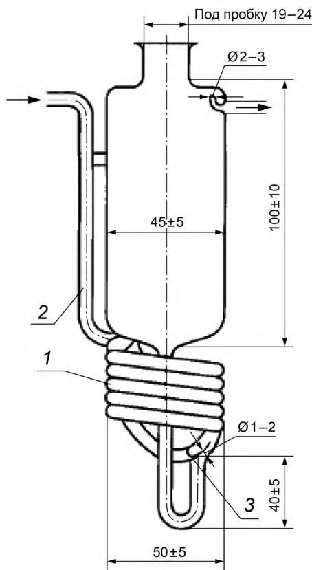
1 — пять полных витков трубки диаметром (6 \pm 1) мм; 2 — стеклянная перегородка; 3 — место впаива газопроводящей линии
