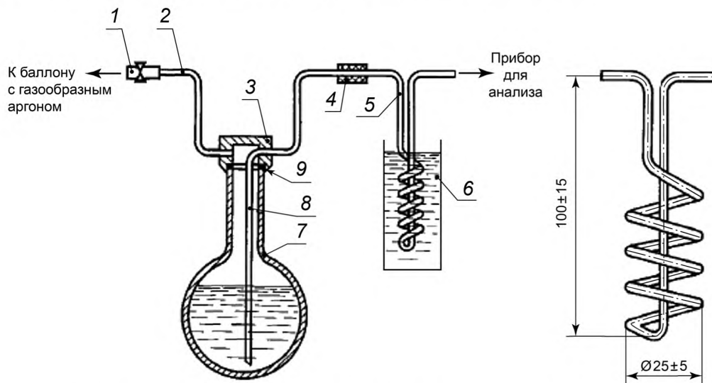
1 — резиновая трубка с зажимом; 2 — медная трубка 6 \times 1 ; 3 — крышка; 4 — резиновая трубка; 5 — змеевиковый испаритель; 6 — сосуд с водой; 7 — криогенный сосуд; 8 — трубка из нержавеющей стали 3 \times 0,7 ; 9 — прокладка
