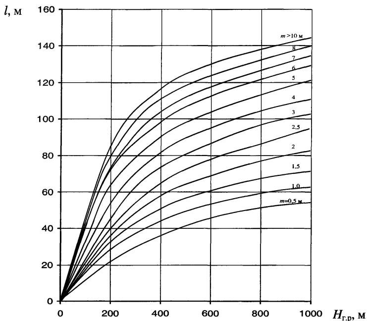
Рис. 2. Номограмма для определения ширины зоны опорного давления:
