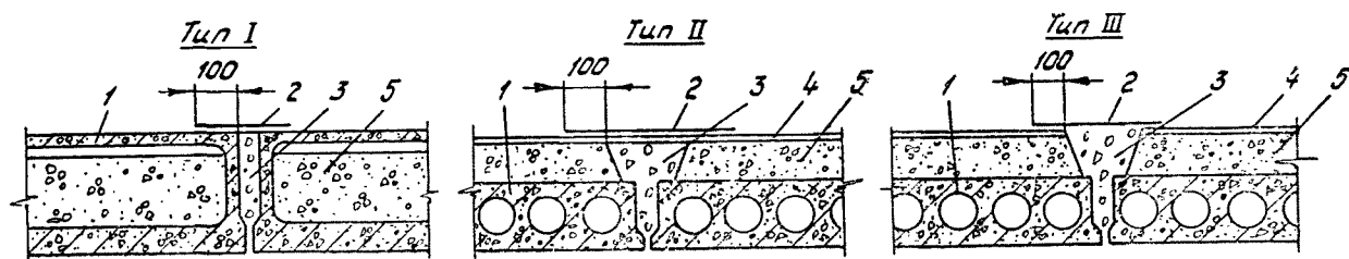
Рис. 2. Типы стыков
