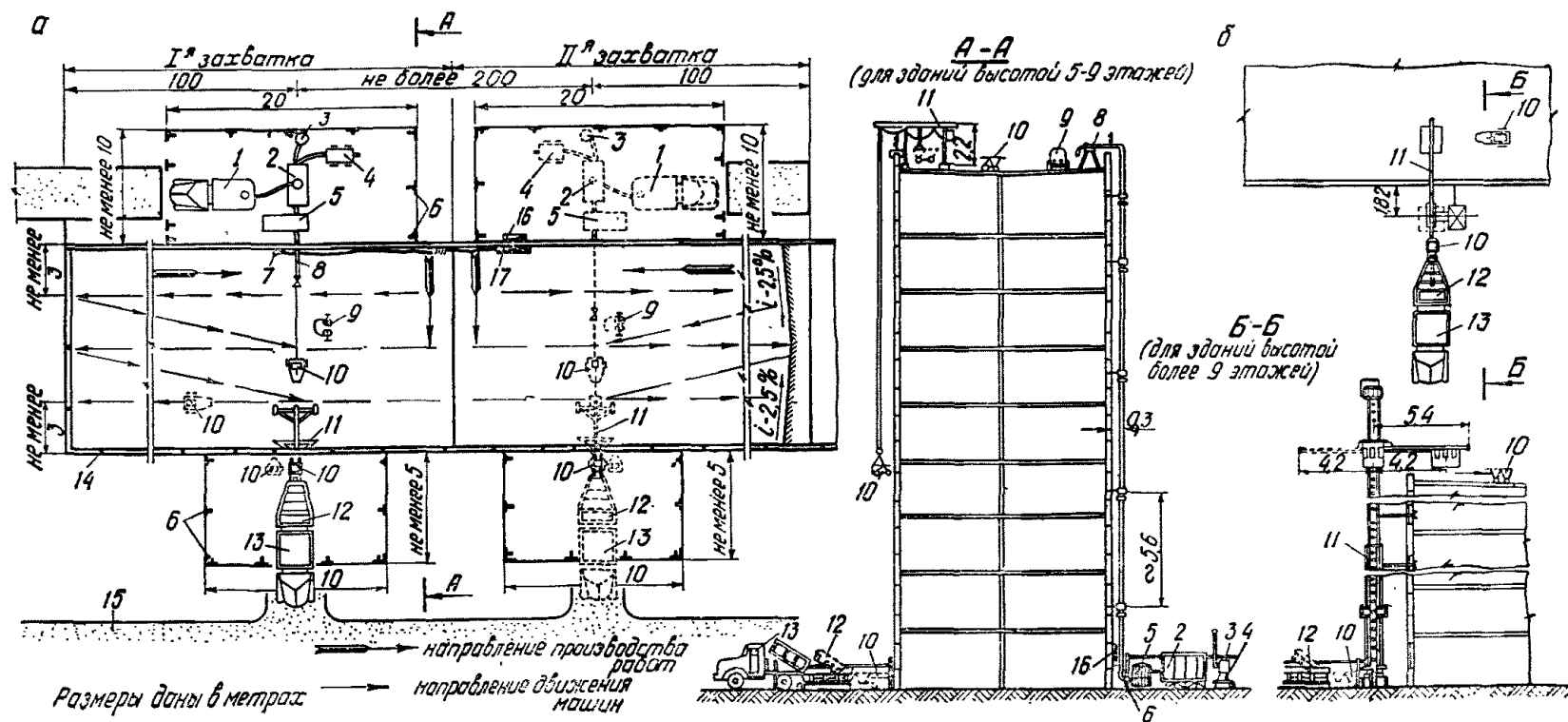
Рис. 1. Схема производства работ при заделке стыков плит покрытия в жилых зданиях
