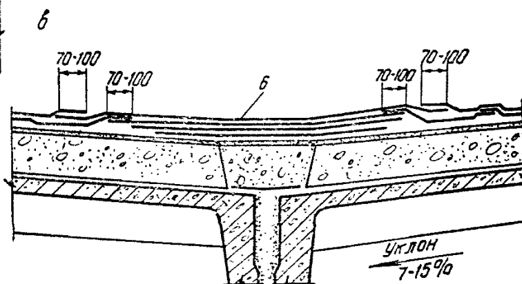
Рис. 8. Детали обделки деформационного шва и ендов
