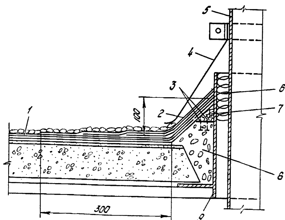
Рис. 6. Устройство гидроизоляционного ковра в местах пропуска труб через стальной патрубок
