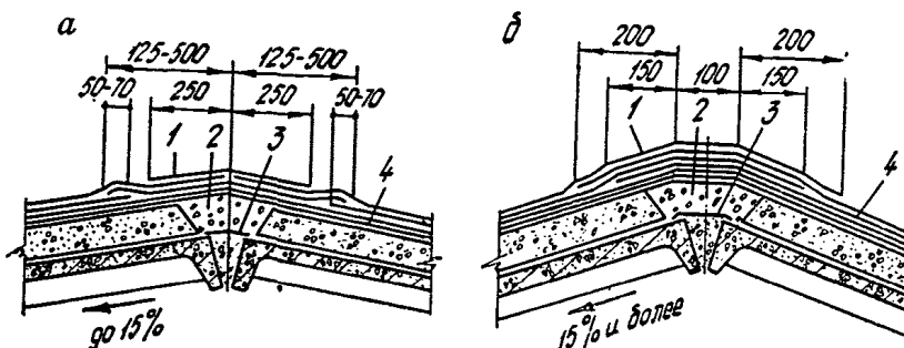
Рис. 3. Покрытие конька
