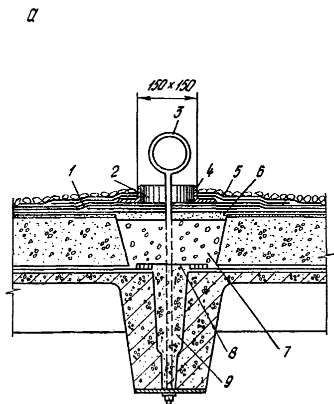
Рис. 9. Устройство гидроизоляционного ковра
