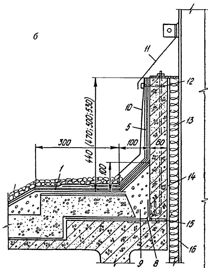
Рис. 9. Устройство гидроизоляционного ковра
