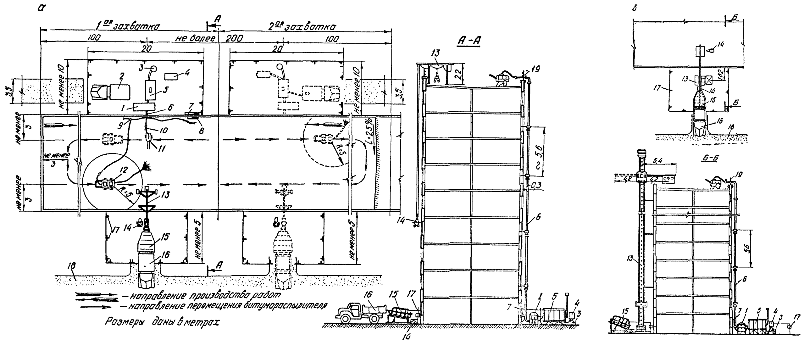
Рис. 2. Схема производства работ
