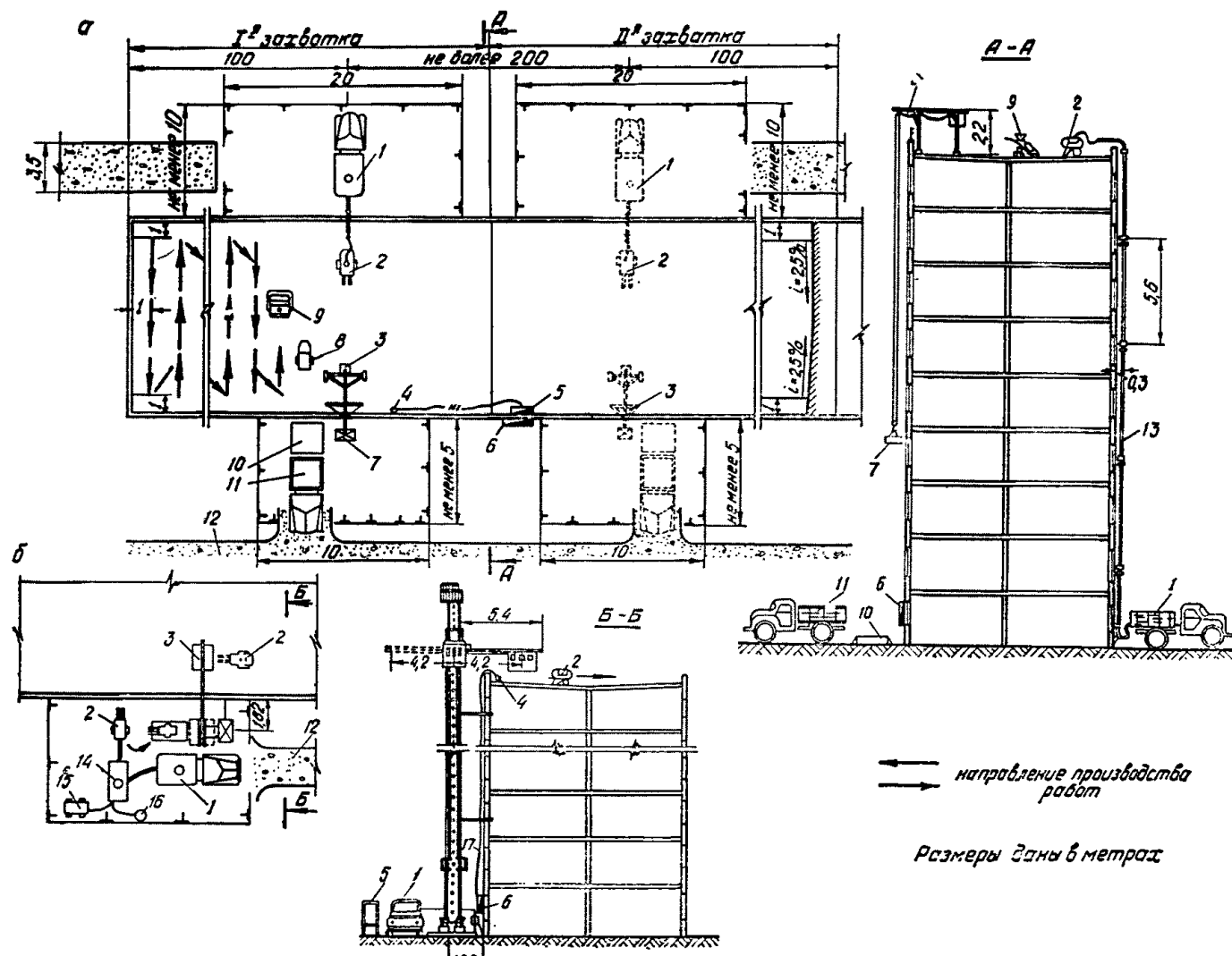
Рис. 2. Схема производства работ
