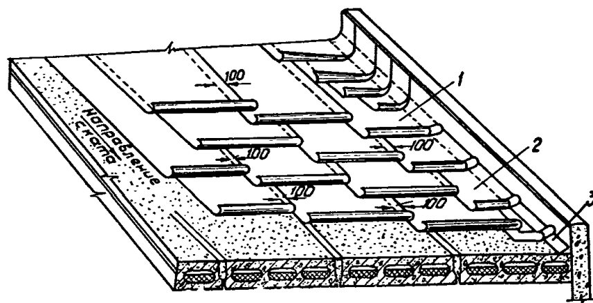
Рис. 3. Деталь устройства четырехслойного рулонного ковра в местах примыканий
