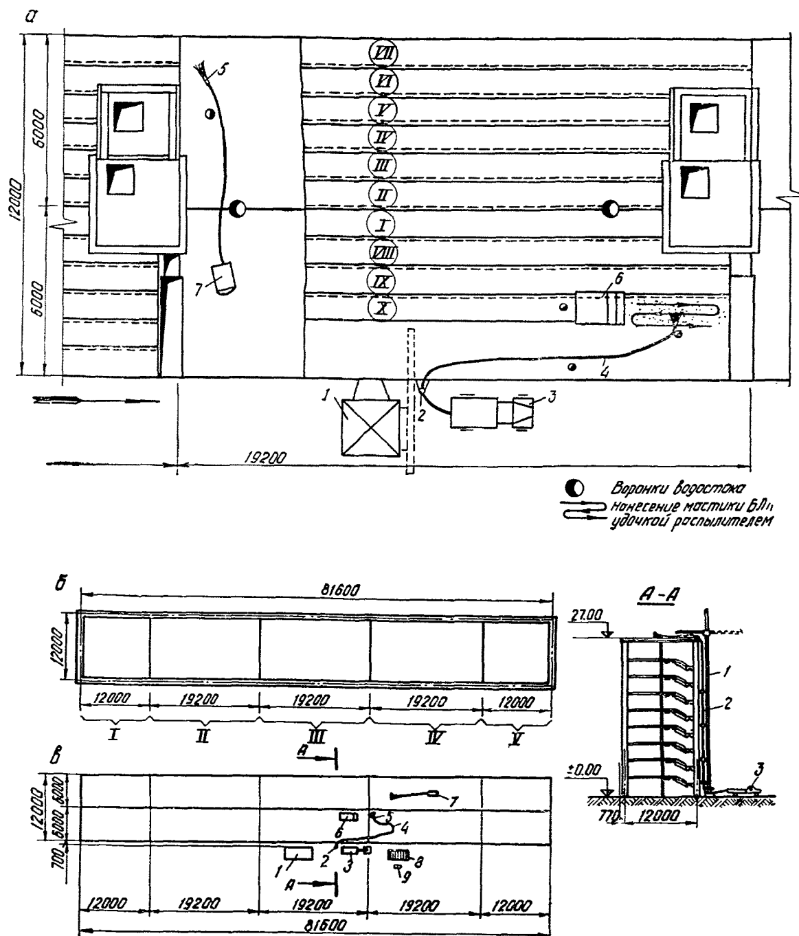
Рис. Схема устройства гидронизоляционного ковра
