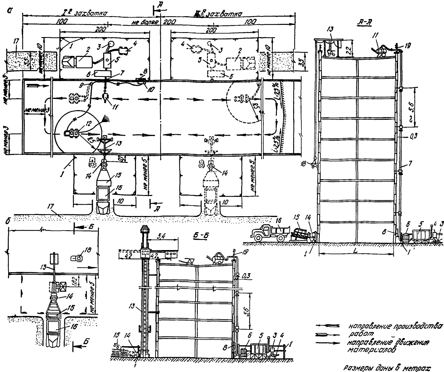
Рис. 2. Схема производства работ
