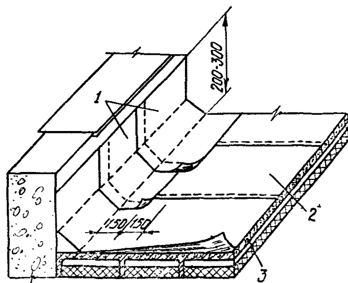
Рис. 4. Схема устройства гидроизоляционного ковра в местах примыканий
