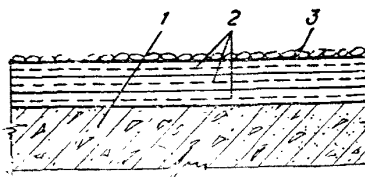
Рис. 1. Схема конструкции трехслойной мастичной кровли.
