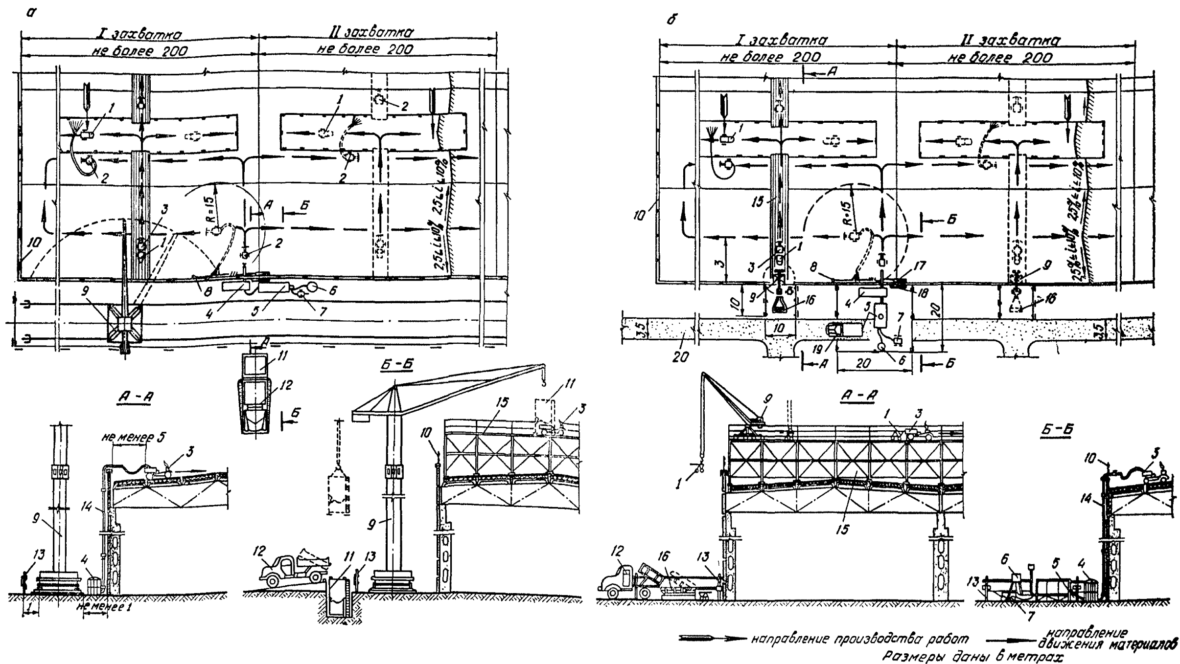
Рис. 2. Схема производства работ
