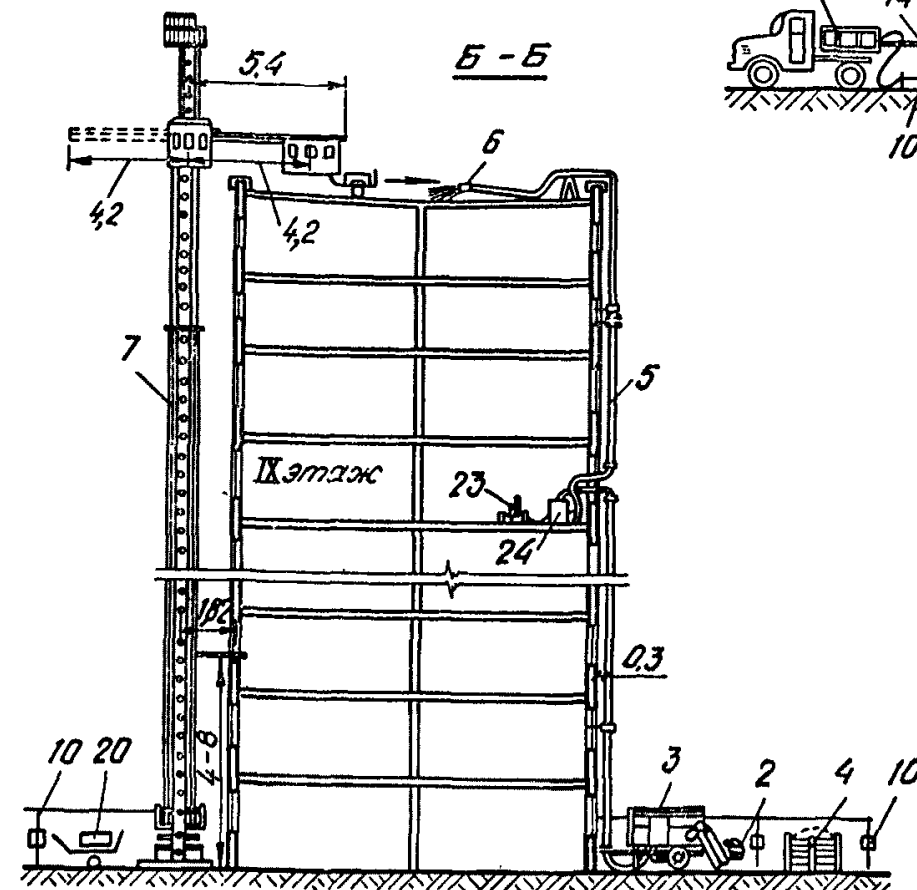
Рис. 2. Схема производства работ
