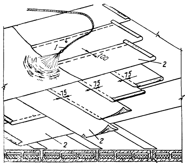
Рис. 3. Схема устройства кровли из битумной мастики эмульбита, армированной тремя слоями стеклохолста
