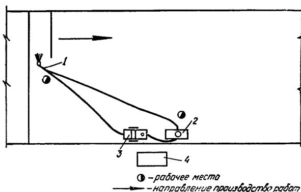
Рис. Устройство защитного слоя краской БТ-177 — пистолет-распылитель; 2 — краскопульт; 3 — компрессор СО-2; 4 — подъемник УПС
